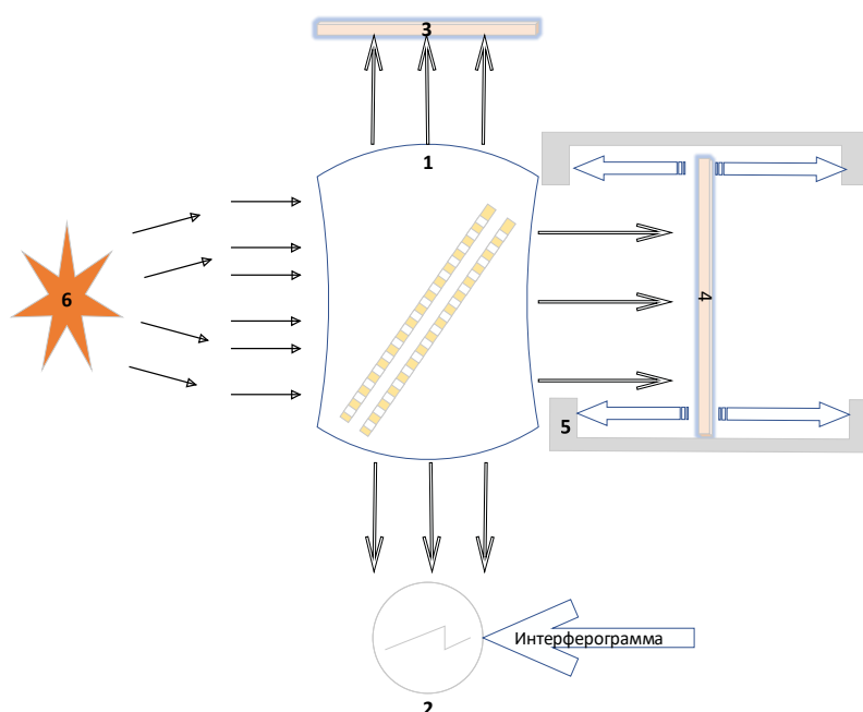
Рис. 2 Принципиальная оптическая схема интерферометра Майкельсона с подвижным зеркалом
