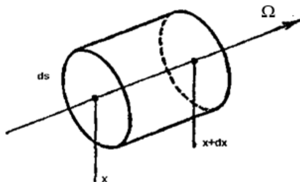
Рис. 3 К выводу уравнения переноса излучения
