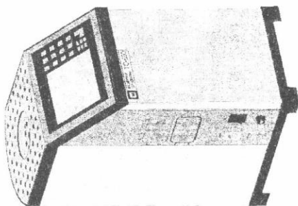
Рис. 4. Портативный калибратор температуры ТС-600
