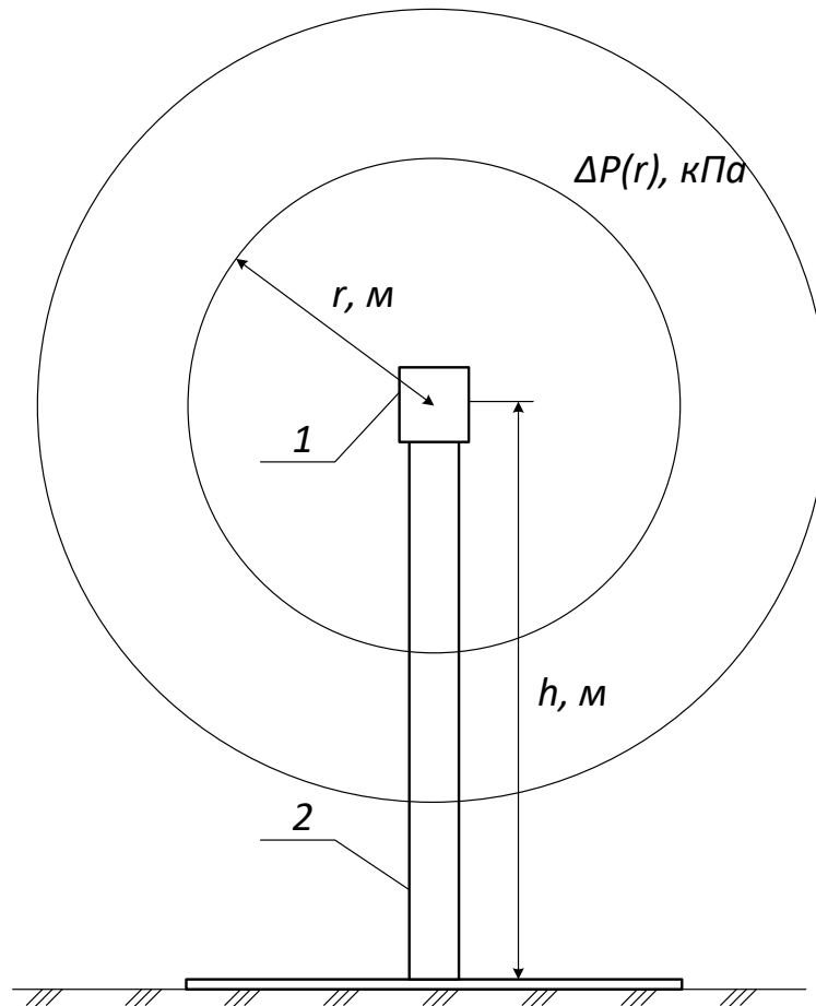
Рисунок 4. Схема факельного стовбуру та розрахункових параметрів вибуху: 1 – факельний оголовок; 2 – факельний стовбур; h – висота факельного стовбуру, м; r – радіус надлишкового тиску вибуху; \Delta P – надлишковий тиск вибуху, кПа
