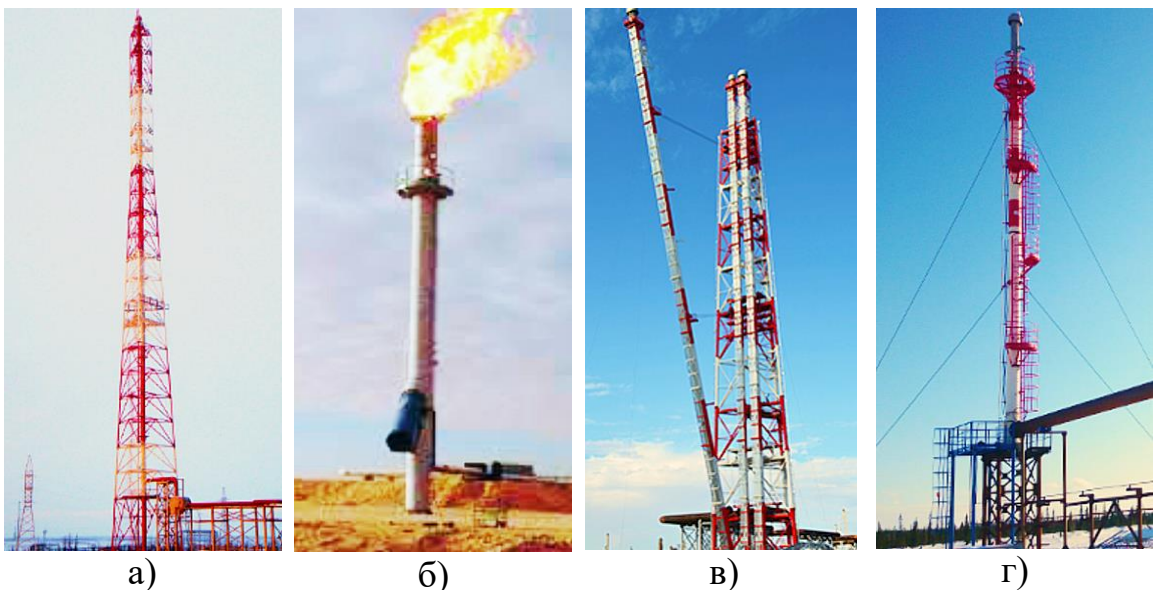
Рисунок 2. Типи факельних стволів: а) щоглові, б) самонесучі, в) з парними стволами, г) на розтяжках
