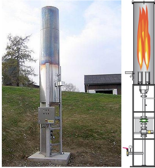
Рисунок 3. Автоматизований факельний пристрій для біогазового комплексу
