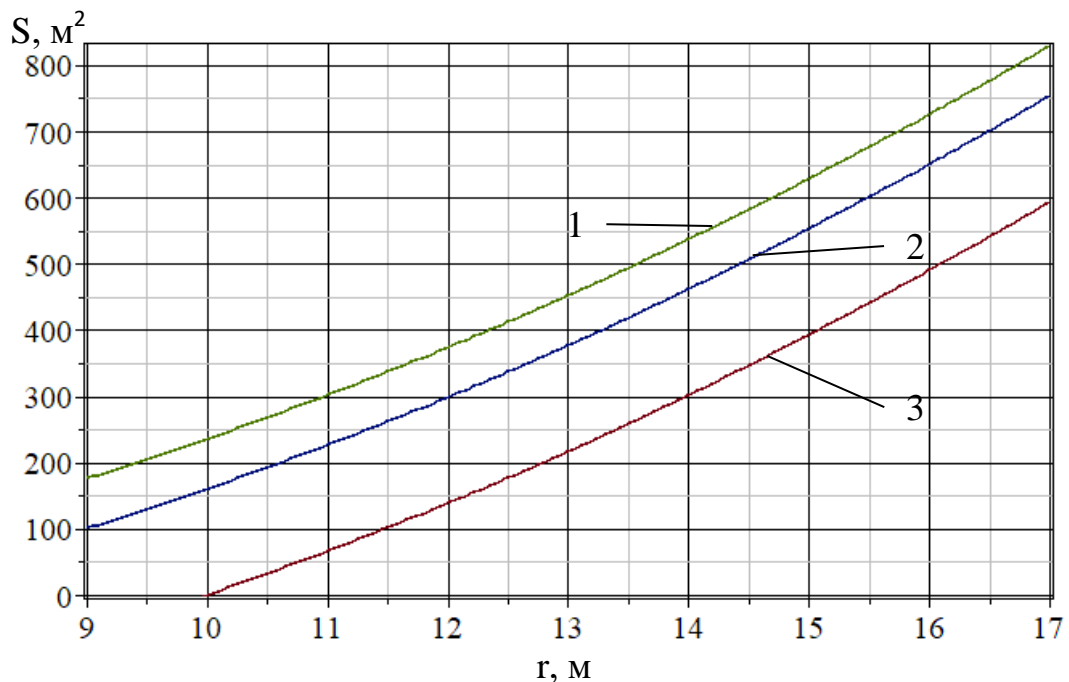
Рисунок 6. Залежність площі, що підпадає під вплив розрахункового надлишкового тиску вибуху, від радіуса при різних висотах факельного стовбуру: 1 – h=5 м; 2 – h=7 м; 3 – h=10 м
