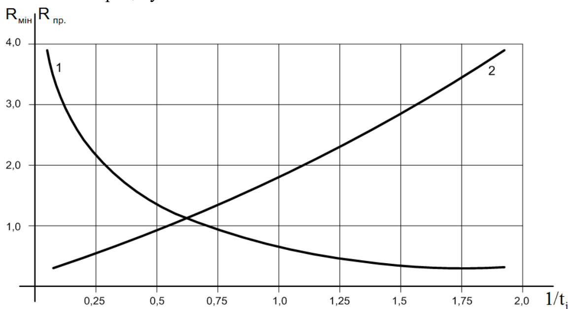
Рис. 5 – Аналітичні залежності зміни коефіцієнту простою мін ОЗМ-72 R_{мін} (1) та коефіцієнту простою працівників R_{пр.} (2) від часу знаходження міни на i -му етапі (при виконанні i -ої операції)
