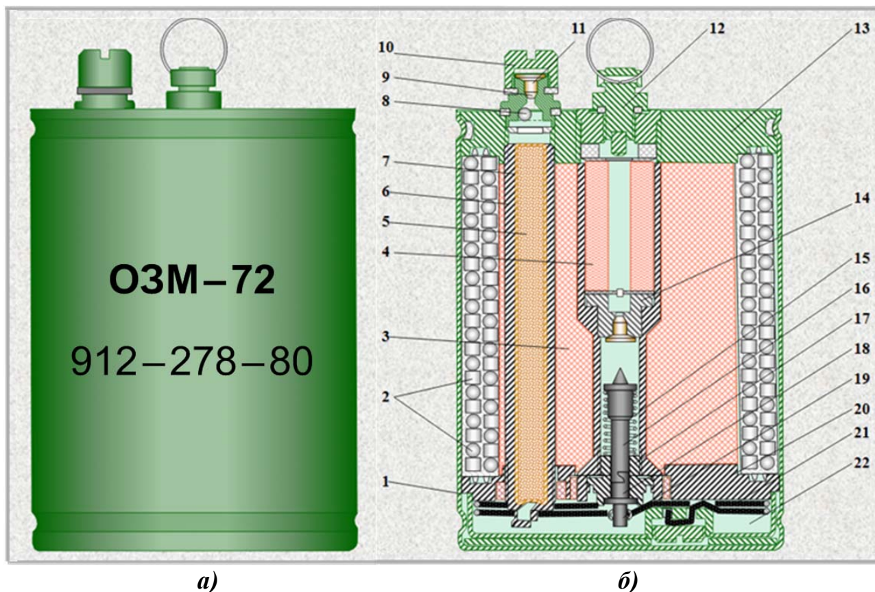
Рис. 1 – Будова протипіхотної осколкової міни, що вистрибує, кругової поразки ОЗМ-72: а) загальний вигляд міни; б) конструкція міни; 1 – направляючий стакан; 2 – осколки; 3 – заряд ВР; 4 – додатковий детонатор; 5 – вишибний заряд; 6 – центральна втулка; 7 – трубка; 8 – кулька; 9 – ніпель; 10 – ковпачок; 11 – капсуль-запалювач; 12 – пробка зі скобою; 13 – верхня кришка; 14 – втулка з капсулем-запалювачем; 15 – пружина; 16 – ударник; 17 – втулка; 18 – п’ятка ударника; 19 – запобіжний ковпачок; 20 – нижня кришка; 21 – натяжний трос; 22 – камера
