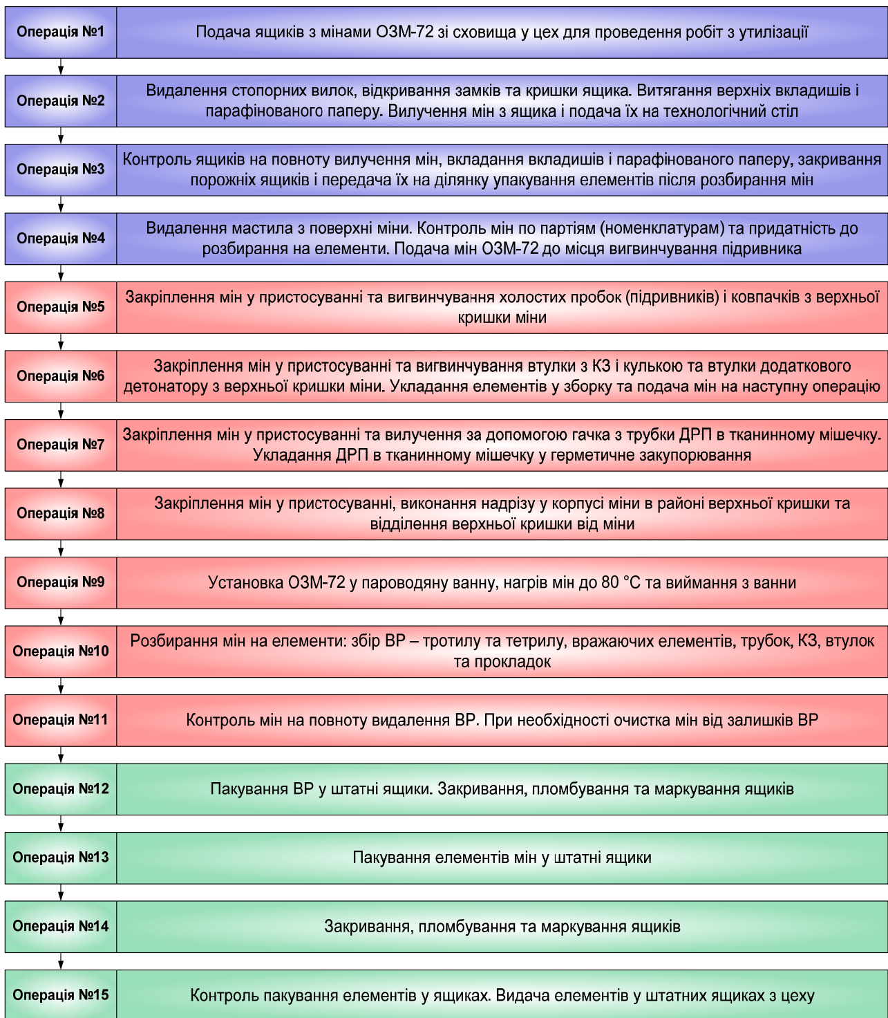
Рис. 2 – Технологічний процес розряджання протипіхотних осколкових мін, що вистрибують, кругової поразки ОЗМ-72
