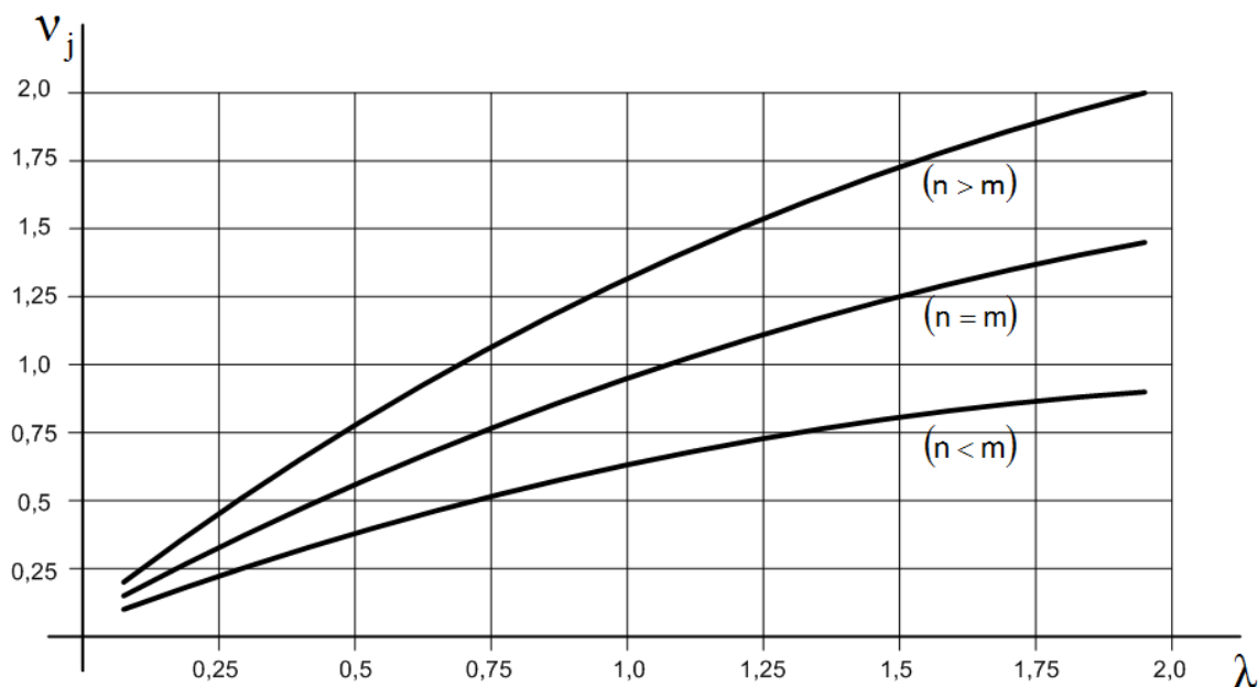
Рис. 4 – Аналітичні залежності між інтенсивністю надходження мін ОЗМ-72 на обслуговування \lambda та інтенсивністю проведення робіт v_j на кожному робочому місці, з урахуванням наявного людського ресурсу
