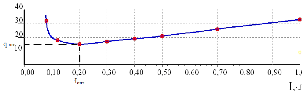
Рис. 2 Залежність питомих витрат води від інтенсивності її подавання на гасіння модельного вогнища пожежі класу А
