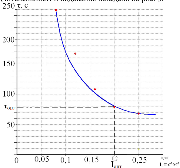
Рис. 3. Залежність часу гасіння модельного вогнища пожежі класу А розпиленою водою від інтенсивності подавання: I_{\text{опт}} – оптимальне значення інтенсивності подавання води; \tau_{\text{опт}} – оптимальний час гасіння;
