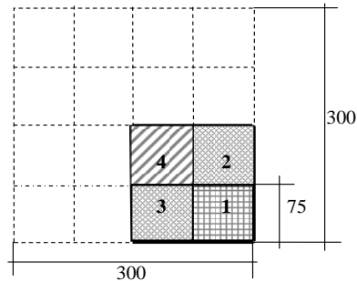
Рисунок 1 - Фізичне розділення перерізу залізобетонної колони на скінченну кількість елементів
