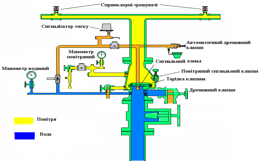
Рисунок 2 Вузол керування повітрязаповненою системою пожежогасіння (повітряний клапан DRV-1)
