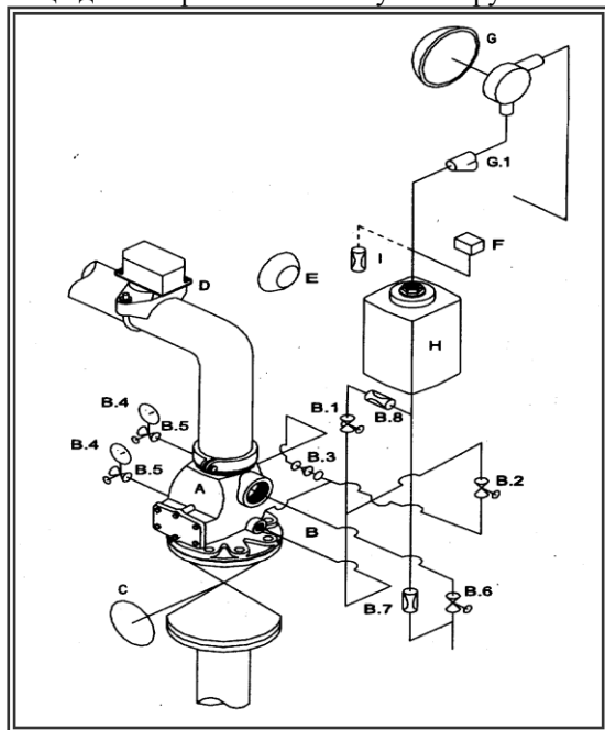
Рисунок 1 Вузол керування водозаповненою системою пожежогашіння (водосигнальний клапан VIKING модель J-1)
