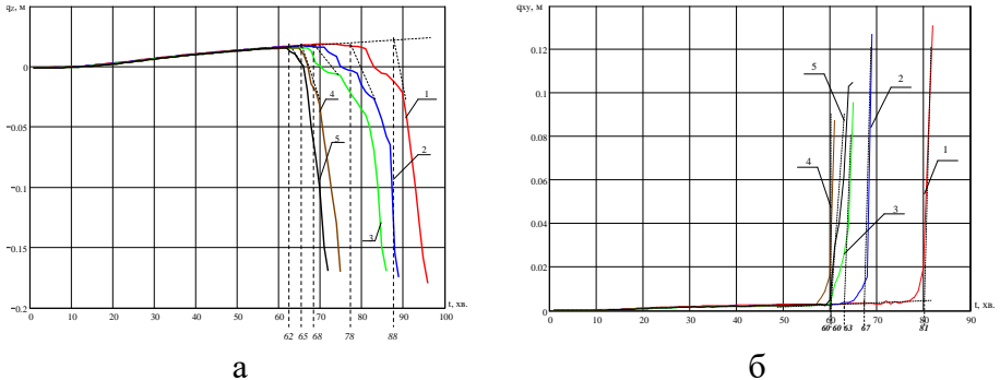
Рисунок 4 - Залежності повздовжніх (а) та поперечних (б) деформацій залізобетонних колон від часу при розрахунку межі вогнестійкості
