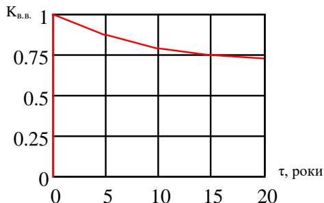
Рисунок 5 - Залежності між вогнестійкості залізобетонних колон від часу впливу агресивних факторів оточуючого середовища (а) та коефіцієнт втрати вогнестійкості залізобетонних колон (б)
