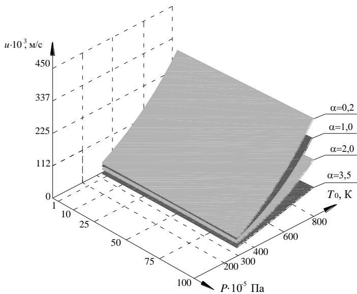
Рис. 3. Тривимірне зображення залежностей швидкості горіння суміші цирконій + нітрат натрію від температури нагріву та зовнішнього тиску для різних значень коефіцієнту надлишку окислювача ( d_M = 5 \text{ мкм} ).
