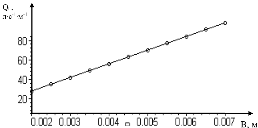
Рисунки 2 – Залежність удельного расхода ОВ от глубины ВЗ
