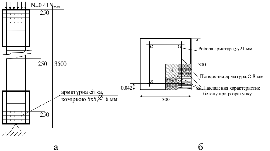
Рисунок 2 - Розрахункова схема колони для проведення розрахунку вогнестійкості за ознакою втрати несучої здатності (а – повздовжній вигляд, б – поперечний вигляд).
