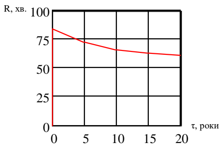
Рисунок 5 - Залежності між вогнестійкості залізобетонних колон від часу впливу агресивних факторів оточуючого середовища (а) та коефіцієнт втрати вогнестійкості залізобетонних колон (б)
