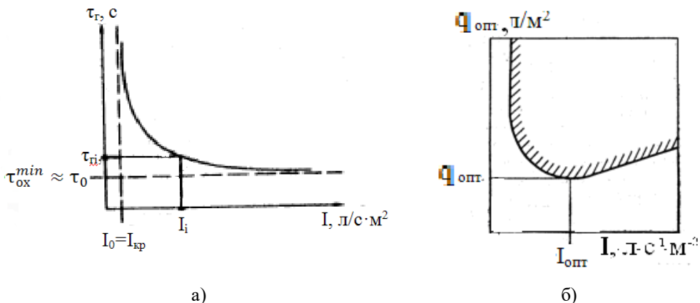
Рис. 1 а) Залежність тривалості гасіння деревини від інтенсивності подавання води, б) Залежність витрат води від інтенсивності її подавання
