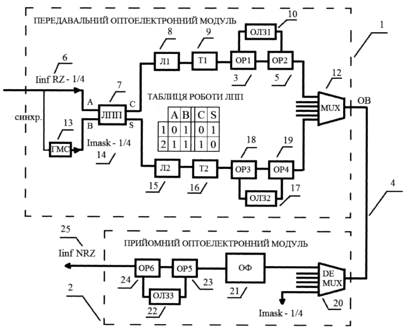
Риунок 1 Пристрій маскування конфіденційної інформації
