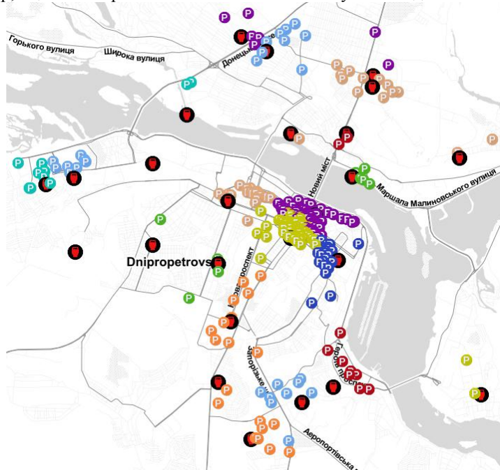
Рис. 1. Оптимальне розміщення 25 зарядних станцій у місті Дніпро
