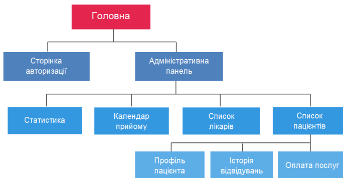
Рисунок 1 – Структура сторінок
