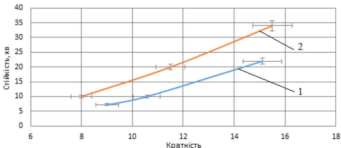
Рисунок 7 – Залежність стійкості піни від кратності для різних режимів генерування піни. Тиск у передкамері установки 0,8 МПа, 1 – 5% водний розчин піноутворювача «БАРС 1S», 2 – 5% водний розчин піноутворювача «БАРС 1S» з добавкою 1% полівінілового спирту
