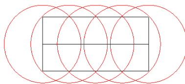
Рис. 4 – Зоны действия пожарных кранов диаметром 65 мм, с рукавами длиной 10 м, стволами с насадками диаметром 13 мм
