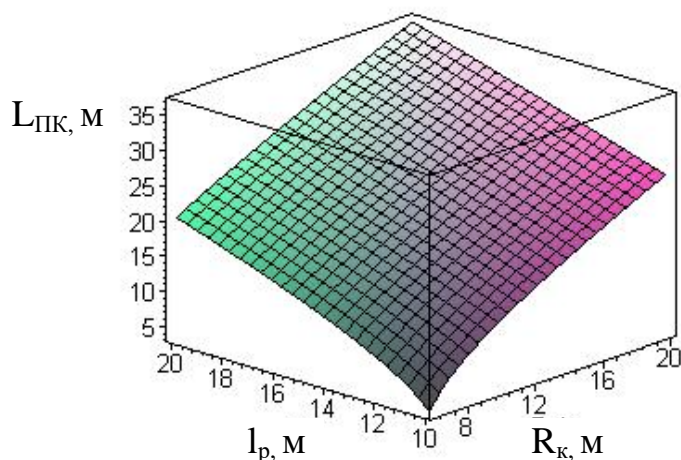
Рис. 3 – Зависимость расстояния между ПК L_{ПК} от длины рукава l_p и радиуса компактной части струи R_k
