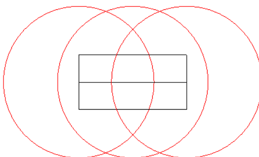
Рис. 5 – Зоны действия пожарных кранов диаметром 65 мм, с рукавами длиной 20 м, стволами с насадками диаметром 19 мм
