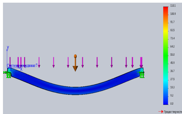
Рисунок 8 – Розподіл навантаження і напруження на балці при підйомі вантажу масою 800 кг
