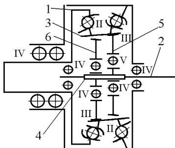
Рис. 7. Структурная схема новой конструкции ВПМ ПТК
