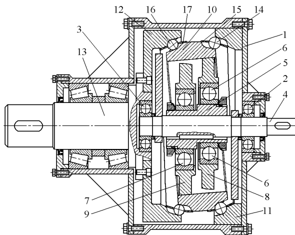
Рис. 6. Конструкция ВПМ ПТК
