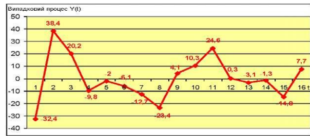
Рис. 3. Графік реалізації випадкового процесу після вилучення систематичної складової зміни надзвичайних ситуацій природного характеру
