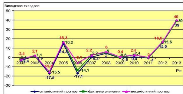
Рис. 12. Значення випадкової складової і прогнозні її значення
