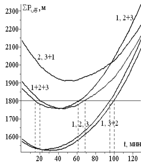
Рис. 2 – Динамика суммарного периметра объединения выпуклых оболочек
