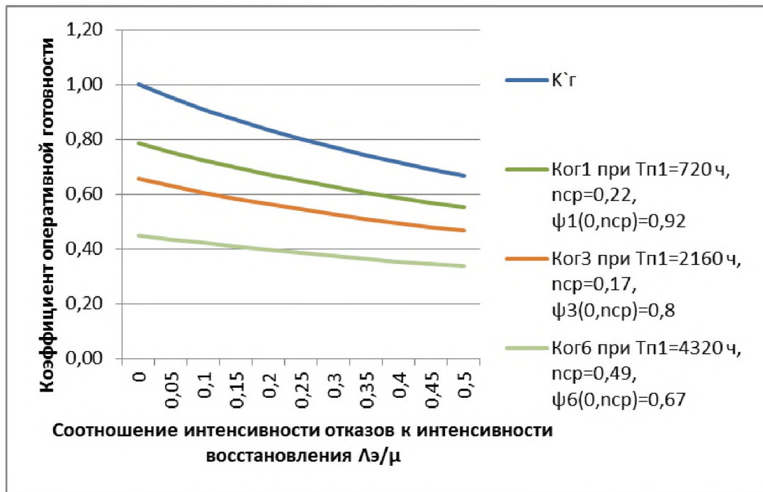
Рисунок 1 – График коэффициента оперативной готовности K_{ог} в дежурном режиме ( K_p = 1 ) в условиях ЧС, при N=100 ; T_{п1} = 720 ч, 2160, 4329 ч; \lambda_э=10^{-6} ч -1
