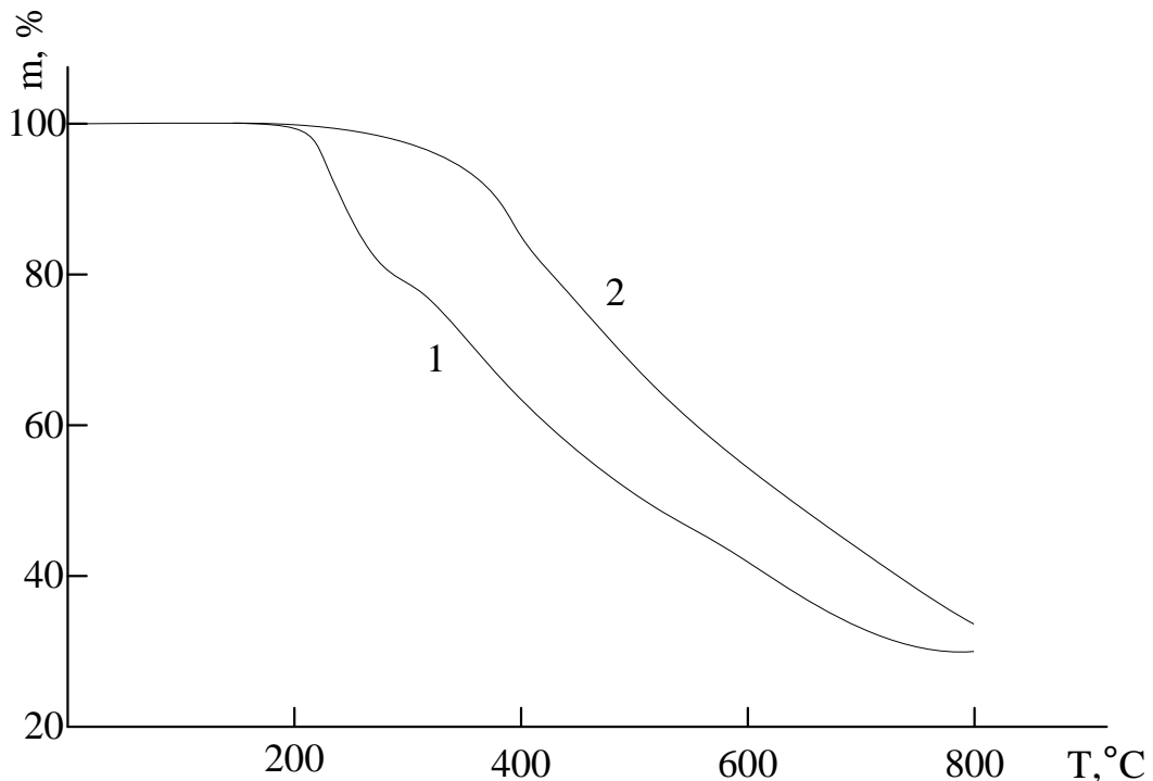
Рис. 1 Дані ТГ волокна нітрон в середовищі аргону (1) та повітря (2).
