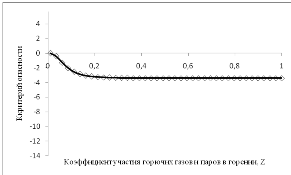
Рис. 4. Критерий R-ukr с изменением коэффициента Z для массы газа 700кг.
