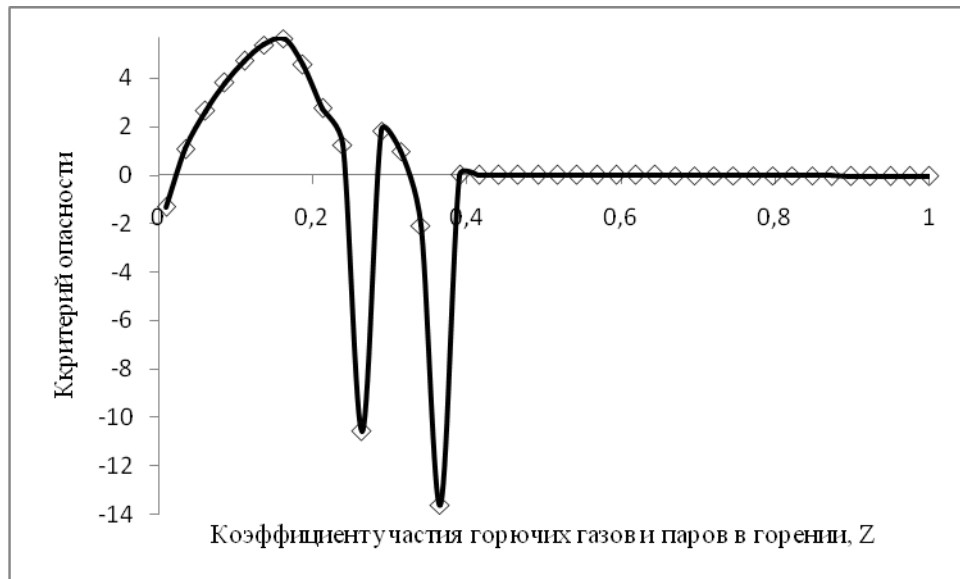
Рис. 5. Критерий R-ukr с изменением коэффициента Z для массы газа 15кг.
