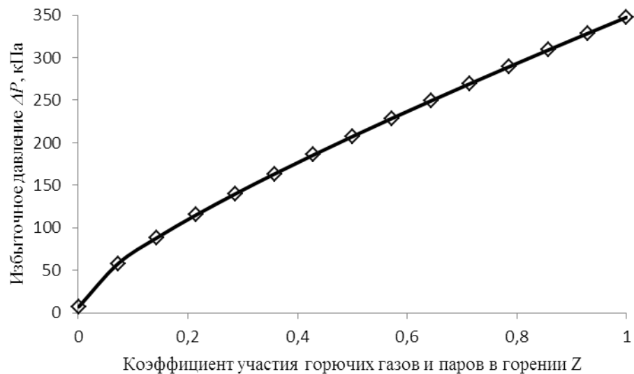
Рис. 1. Изменение избыточного давления с изменением коэффициента Z.
