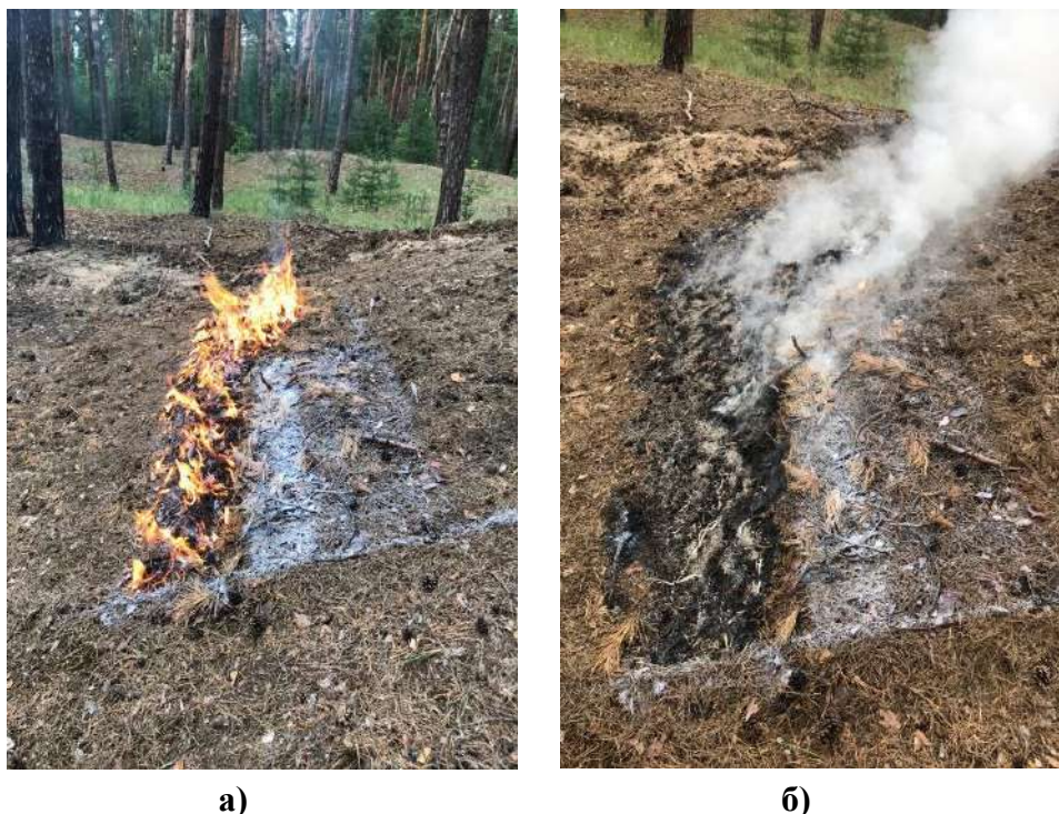
Рис. 2. Зовнішній вид лісової хвойної підстилки: а) під час проведення дослідження; б) після закінчення експерименту
