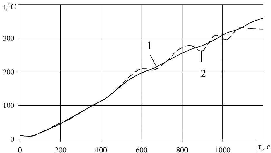
Рис. 1. Залежність температури від часу в місцях вимірювання температур для сталевієї пластини з покриттям: крива 1 – точна крива на необігрівній поверхні; 2 – крива з похибками 10%
