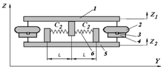
Рис. 2. Схема модифікованого пружного елемента другої ступені пневматичного підвішування із коректором жорсткості. 1 – вантажна платформа, 2 – гумовокордна однофрива оболонка, 3 – дросельна шайба, 4 – додатковий резервуар, 5 – опорна платформа, 6 – пружини коректора жорсткості.
