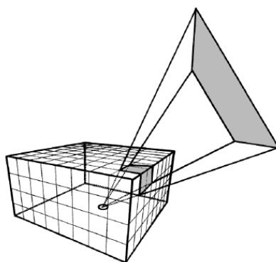
Рис. 1. Геометрична ілюстрація методу пів куба.
