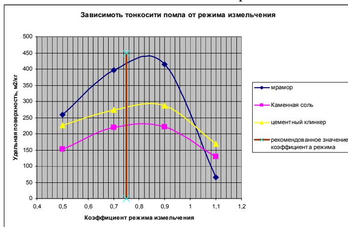
Рис. 1. Зависимость тонкости помола от режима измельчения материала в шаровой мельнице
