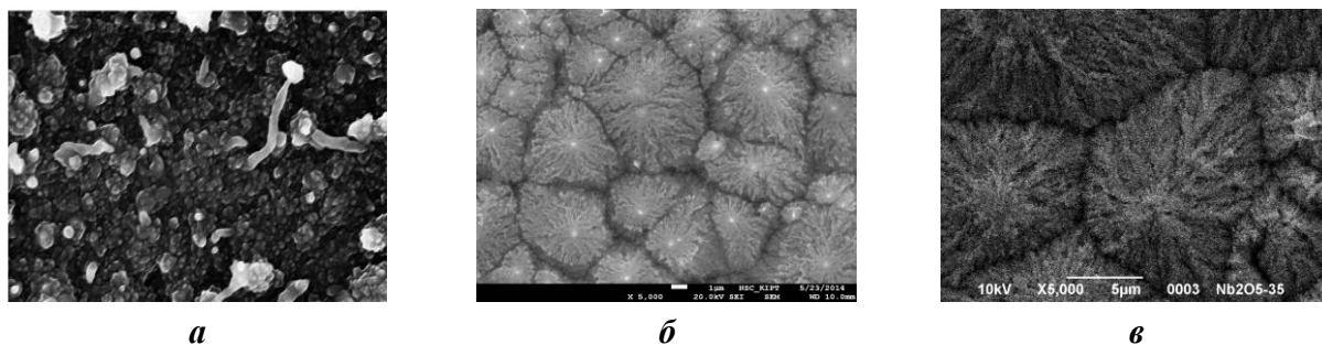
Рис. 1. СЕМ-обстеження поверхні з синтезованим ПАН: а) протонований ПАН емеральдинової форми; б) ПАН оксидних покриттів, синтезованих на ніобії за 60 В у розчині 1М H 2 SO 4 +0,5М NaF упродовж 2 год.; в) АОП ПАН на ніобії в розчині 1М H 2 SO 4 +0,5М NaF упродовж 5 год.
