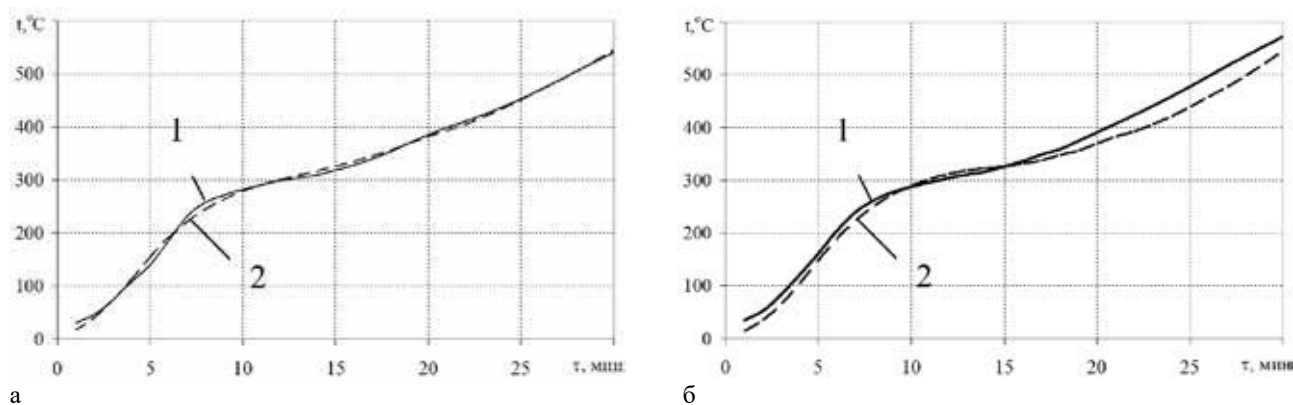
Рис. 6. Зависимость температуры от времени огневого воздействия на необогреваемой поверхности образца с покрытием (а – для комбинаций термопар Т2-Т3 и Т1-Т3; б – для комбинаций термопар Т2-Т1): 1 – полученная по результатам испытаний на огнестойкость 2 – расчетная кривая, полученная решением ОЗТ.
