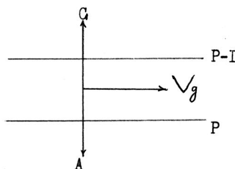
Рисунок 5.8 – Геострофічний вітер:
