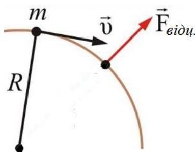
Рисунок 5.6 – Відцентрова сила
