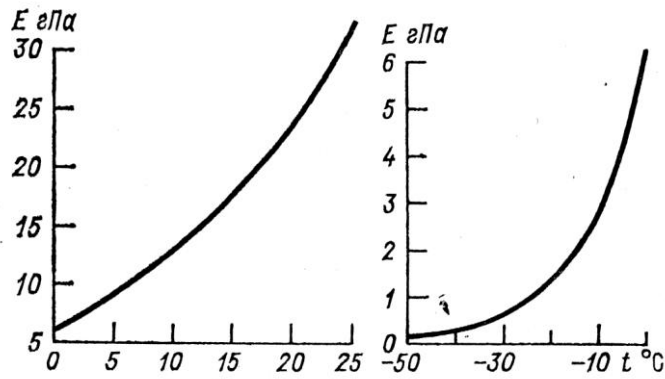
Рисунок 2.4 - Тиск насиченої водяної пари залежно від температури
