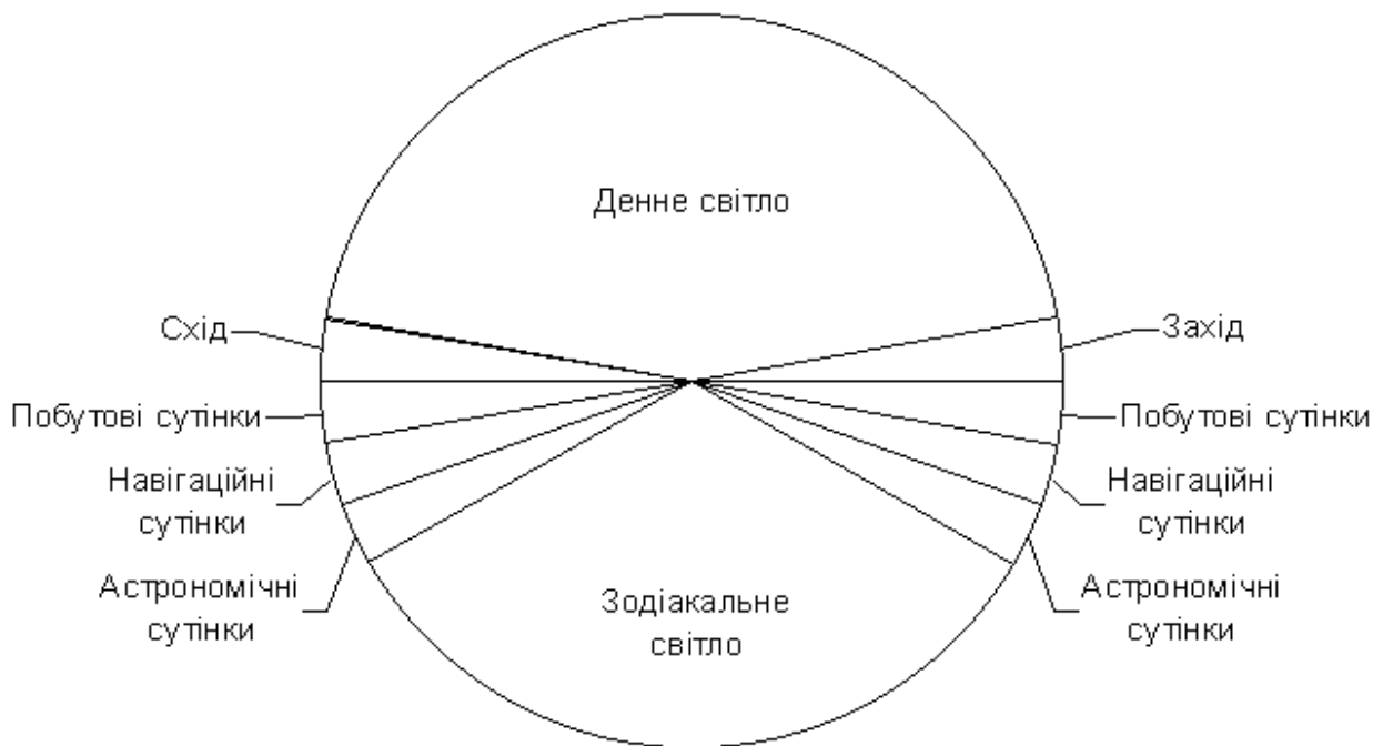
Рисунок 9.4 - Сутінки
