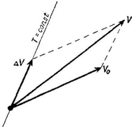
Рисунок 5.10 – Термічний вітер:
