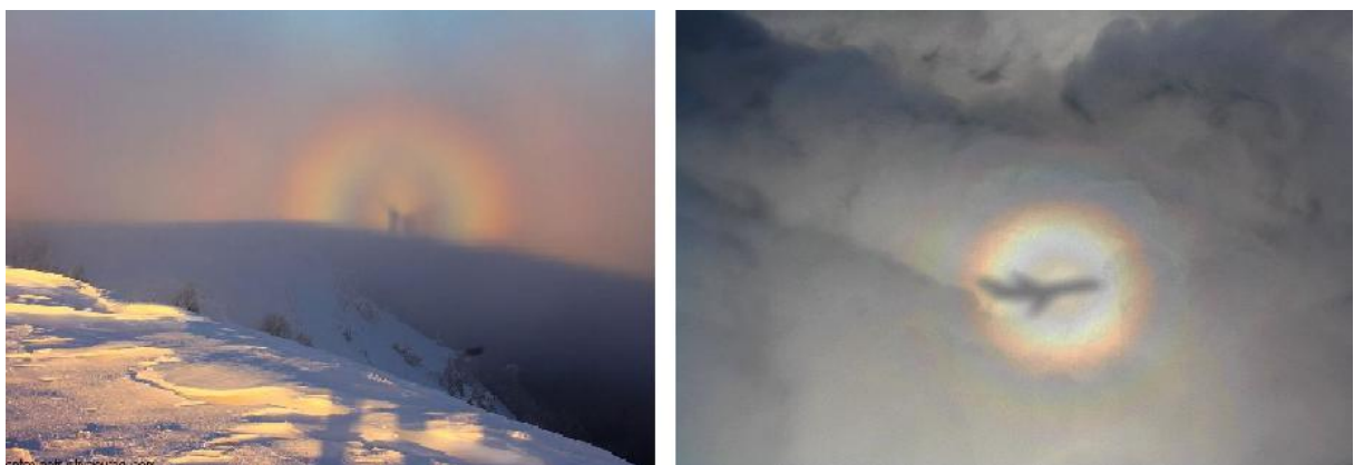
Рисунок 6.10 - Глорія
