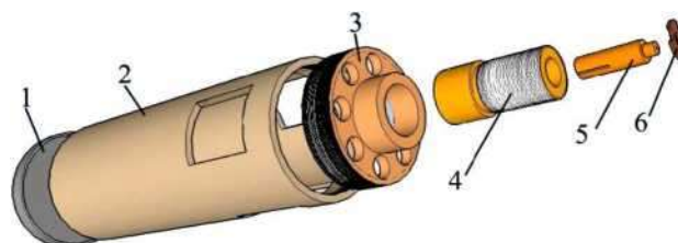
Рис. 1. Основні елементи піногенератора: 1) сітка 05 ГОСТ 3826; 2) стакан; 3) направляюча; 4) корпус; 5) розпилювач; 6) шайба
