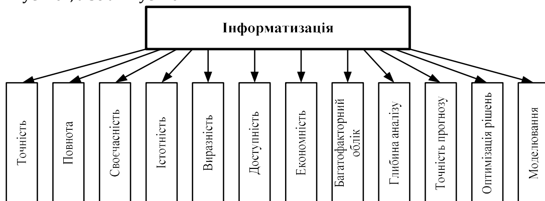
Рисунок 1 – Інформатизація
