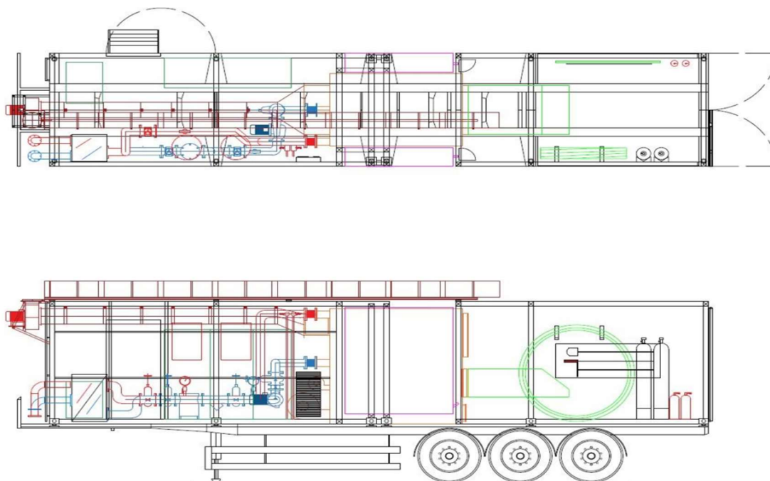
Рисунок 1 – Схема котельні твердопаливної мобільної комплектної
