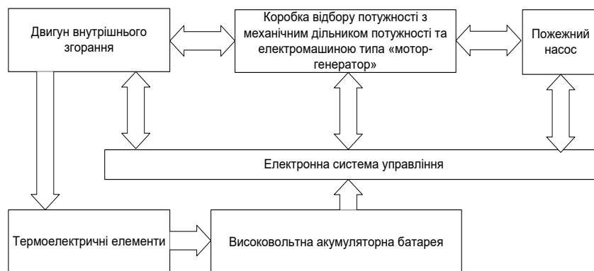
Рис. 1. Загальна схема гібридної силової установки пожежного насоса
