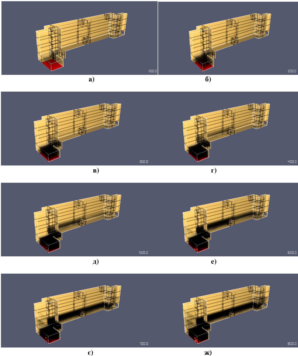
Рис. 14. Візуалізація розповсюдження диму у моделі школи протягом 800 с моделювання: а – 100 с; б – 200 с; в – 300 с; г – 400 с; д – 500 с; е – 600 с; є – 700 с; ж – 800 с
