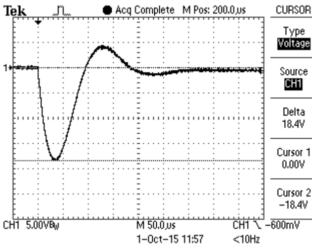
Рис. 13. Осциллограмма импульсной A - компоненты тока имитируемой молнии, воздействующей в сильноточной разрядной цепи высоковольтного генератора ГИТ-А на плоский тонкостенный ИО стальной кровли толщиной h=1 мм ( I_{mA} \approx -192 кА; t_{mA} \approx 34 мкс; \tau_{pA} \approx 500 мкс; J_A \approx 1,9 \cdot 10^6 А 2 ·с)
