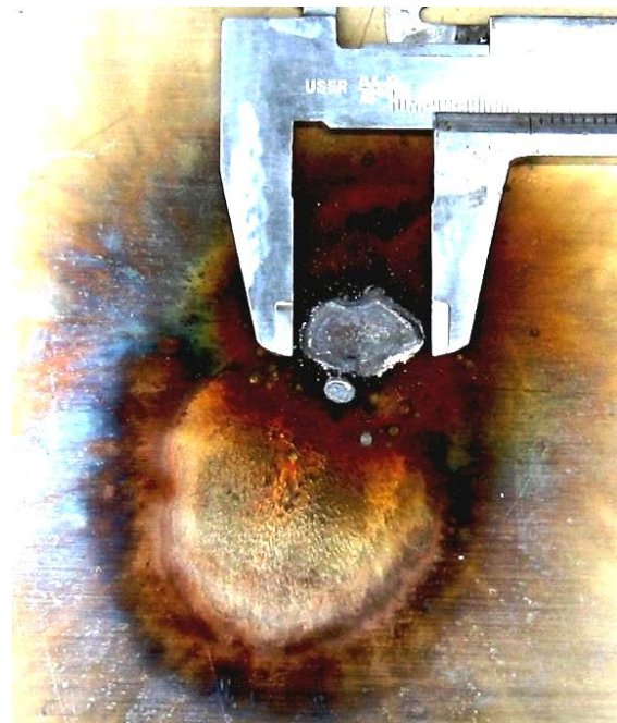
Рис. 8. Общий вид на наружной поверхности ИО стальной кровли округлого очага прямого воздействия на него импульсной A - и длительной C - компонент тока искусственной молнии с нормированными согласно требований [3,4] АВП
