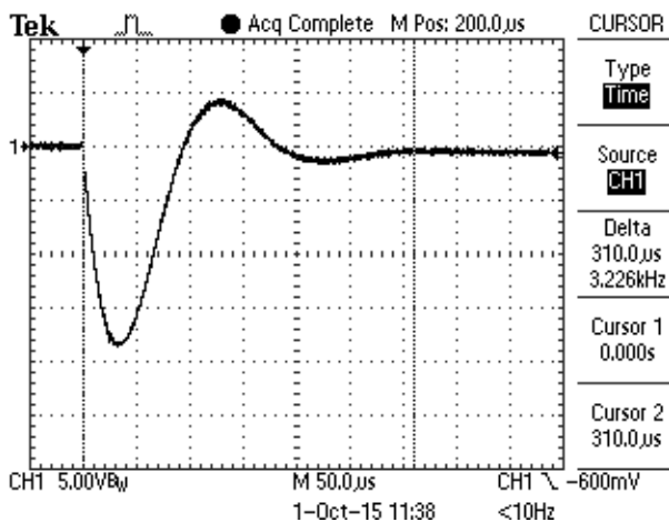
Рис. 10. Осциллограмма импульсной A - компоненты тока искусственной молнии, воздействующей в сильноточной
