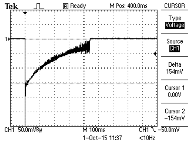
Рис. 11. Осциллограмма длительной C - компоненты тока искусственной молнии, воздействующей на плоский ИО стальной кровли толщиной h=1 мм ( I_{mC}\approx -804 А; t_{mC}\approx 9 мс; \tau_{c}\approx 160 мс; \tau_{pC}\approx 0,448 с; q_C\approx -165 Кл; i_{CC}\approx -367 А)
