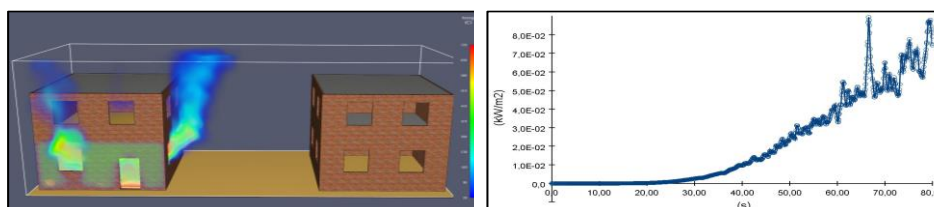
Рис. 1. Приклад моделювання в PuroSim пожежі, визначення теплового потоку від пожежі
