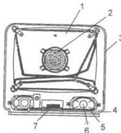
Рис. 1.91. Вид телевізора "Витязь 51 ТЦ 6010" ззаду зі знятим кожухом:
