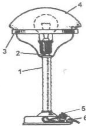
Рис. 1.65. Настільна лампа:
