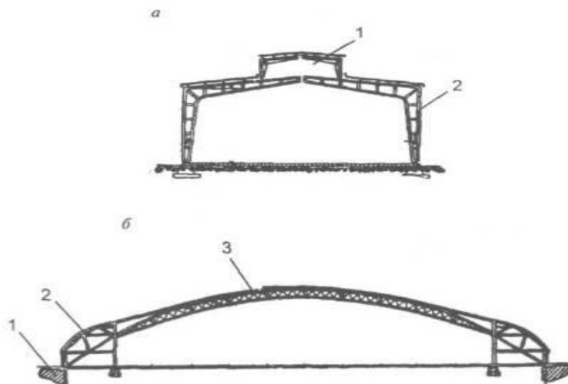
Рис. 1.5. Сталеві несучі конструкції покриттів:
