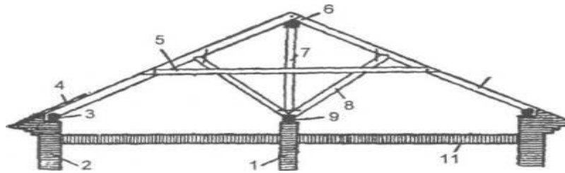
Рис. 1.3. Дерев'яна конструкція з похилими стропилами:
