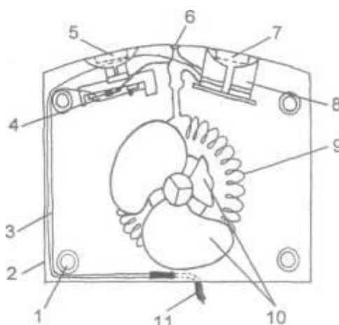
Рис. 1.82. Тепловентилятор Binaton VFH-2405DX (передня кришка знята):
