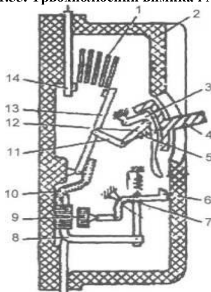
Рис. 1.56. Будова автомата:
