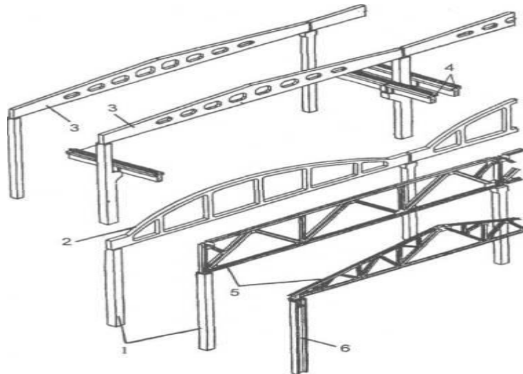
Рис. 1.4. Залізобетонні та сталеві конструкції промислових будівель:
