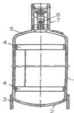
Рис. 1.99. Балон газовий для пропан-бутану (розріз):
