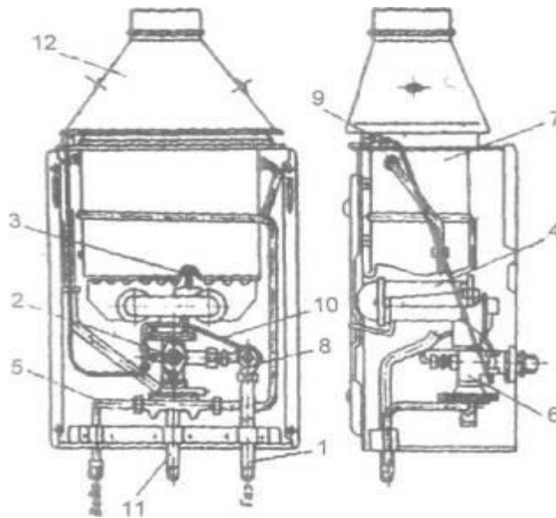
Рис. 1.95. Апарат водонагрівальний проточний газовий побутовий типа ВПГ:
