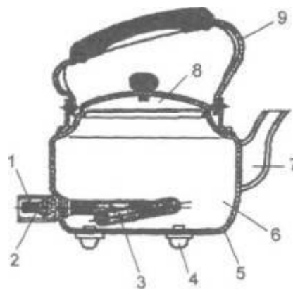
Рис. 1.75. Електричний чайник:
