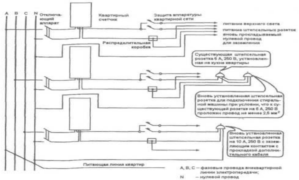
Рис. 1.89. Варіанти підключення автоматичної пральної машини до електромережі
