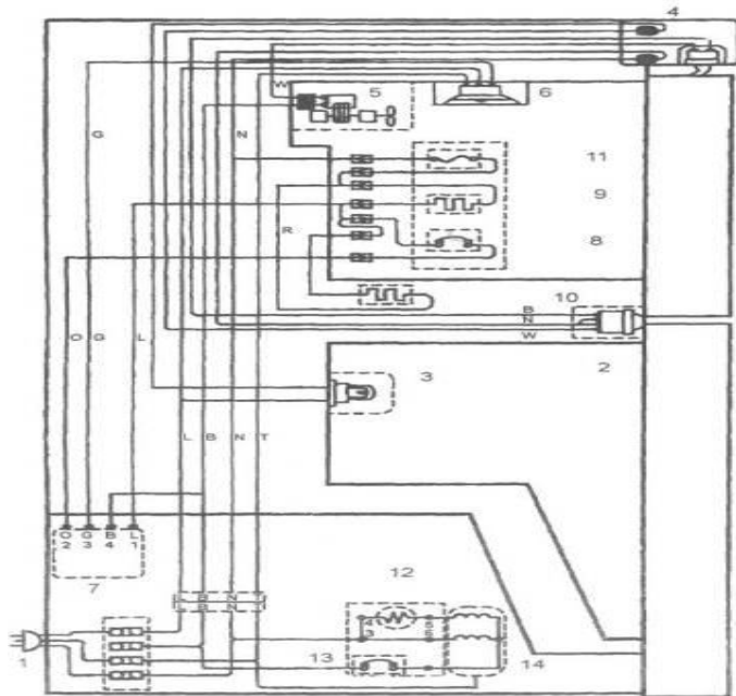
Рис. 1.87. Компонована електрична схема холодильника Ariston:
