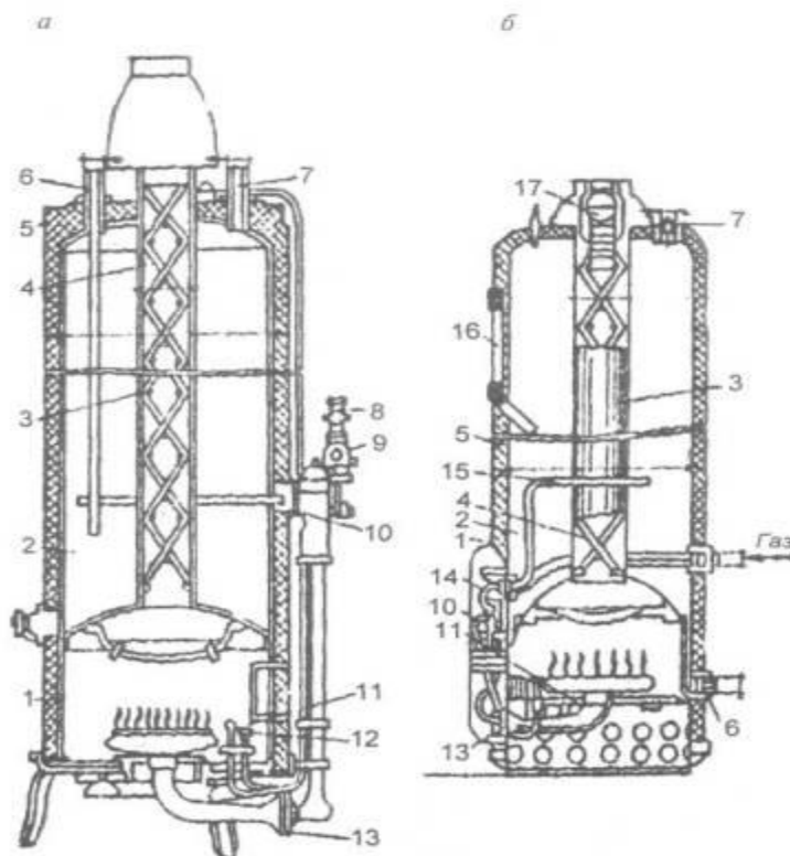
Рис. 1.96. Ємкісні газові водонагрівачі:
