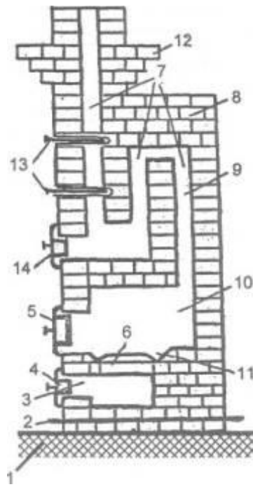
Рис. 1.100. Тепломістка піч:
