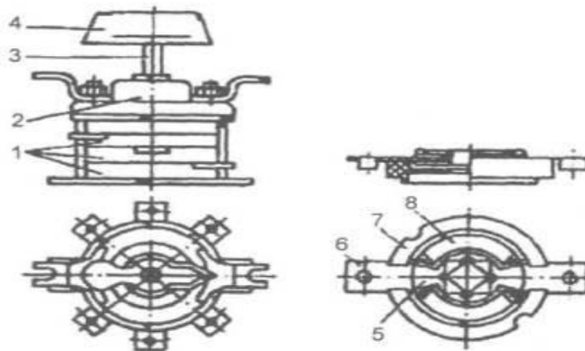
Рис. 1.40. Пристрій пакетного вимикання (перемикач):
