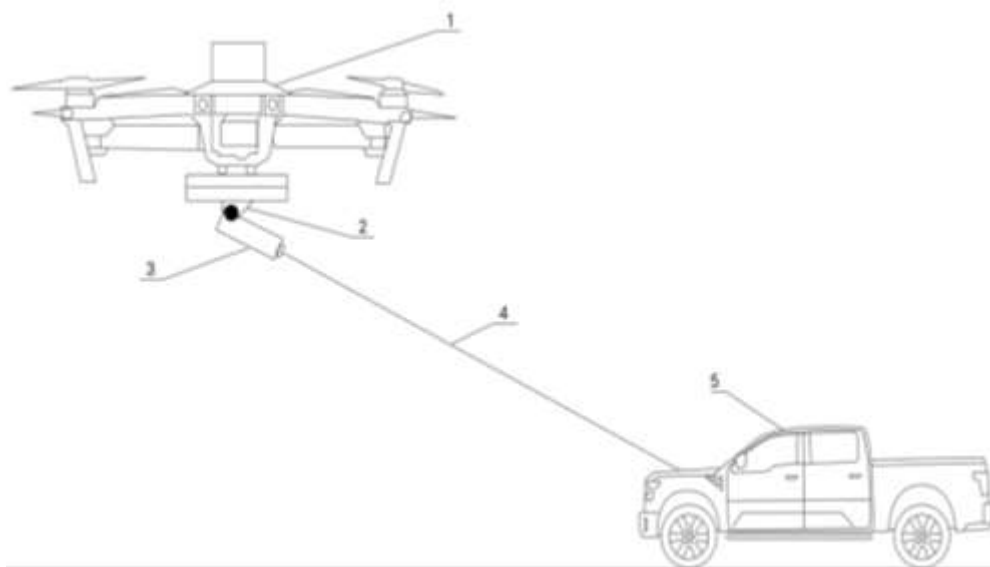
Рис. 1. Дрон з імпульсним квантовим генератором для знешкодження об'єктів ураження
