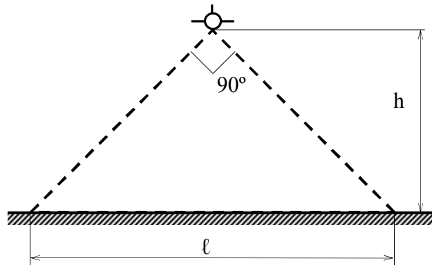
Рис. 1 – Зона огляду фотоапарату БПЛА «Стрепет-С» ( h – висота польоту БПЛА, l – ширина зони фотографування)
