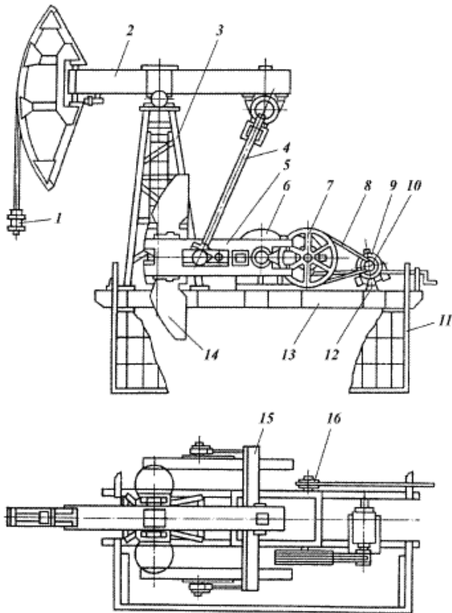
Рис. 16.7 – Станок-качалка:
