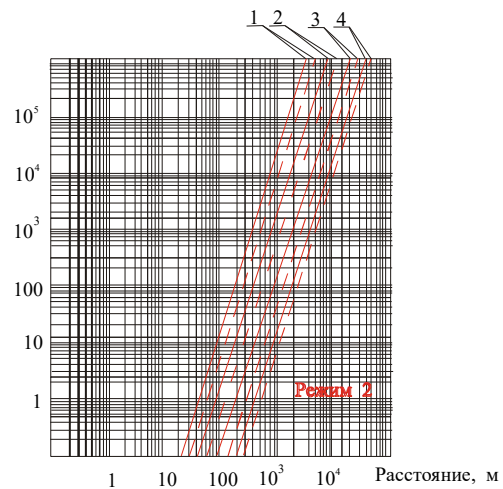
Рисунок 12.3 – Залежність ступеню руйнування будинку від маси палива й відстані:
