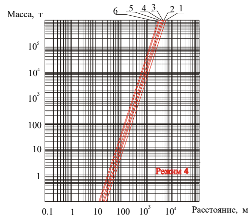
Рисунок 12.11 — Межі зон ураження людей при вибухах хмар ППС:
