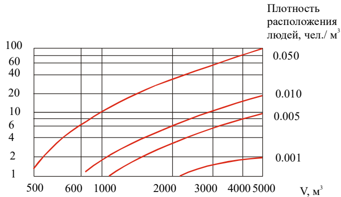
Рисунок 12.17 — исло уражених людей при вибуху посудин високого тиску залежно від об'єму посудини й щільності розташування людей, осіб / м²
