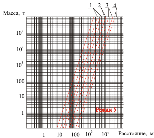
Рисунок 12.6 – Залежність ступеню руйнування будинку від маси палива й відстані:
