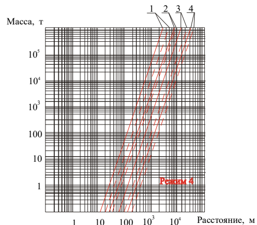
Рисунок 12.5 – Залежність ступеню руйнування будинку від маси палива й відстані:
