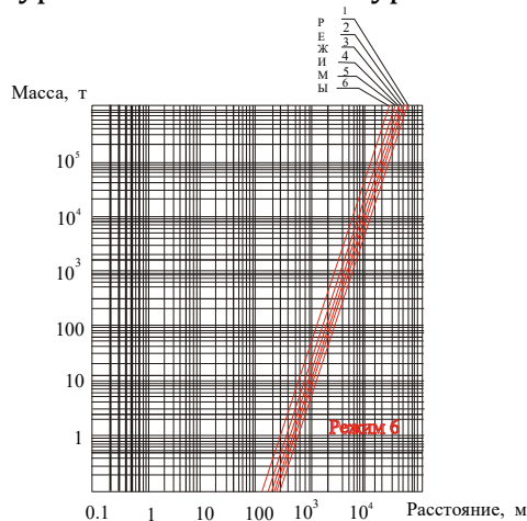
Рисунок 12.14 — Розміри зони руйнування скління при різних режимах вибухового перетворення хмари ППС
