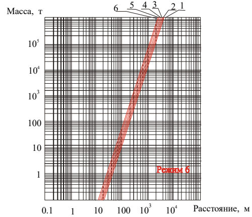
Рисунок 12.13 — Межі зон ураження людей при вибухах хмар ППС:
