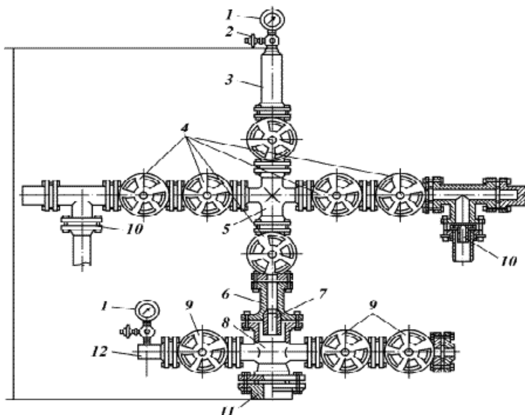
Рис. 16.6 – Арматура фонтанна:
