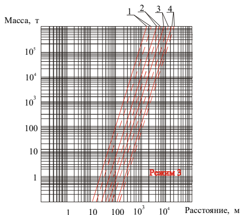
Рисунок 12.4 – Залежність ступеню руйнування будинку від маси палива й відстані:
