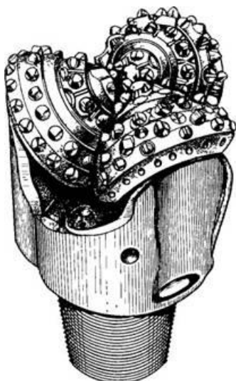
Рисунок 16.5 – Трьохшарошкове долото з вставками з карбіду вольфраму
