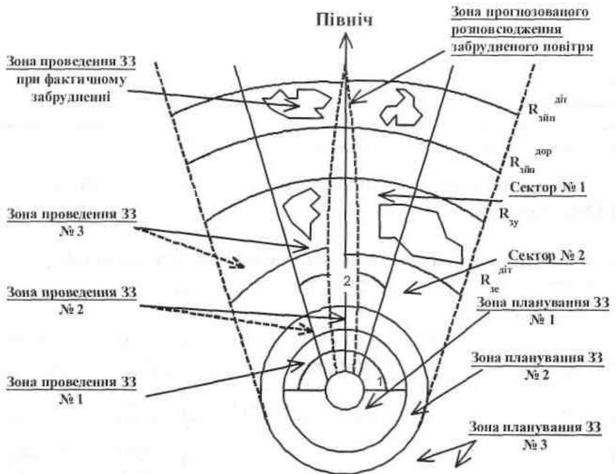
Рисунок 13.2 – Графічне відображення зон планування і проведення заходів щодо захисту населення при аваріях на АС за різними фазами аварії
