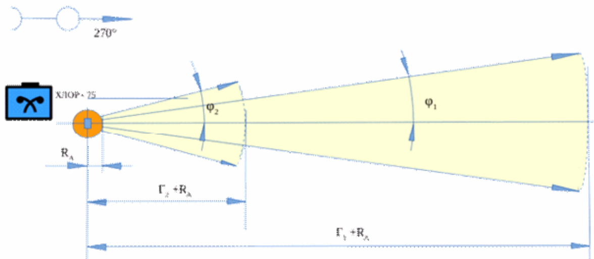
Рисунок 13.1 – Схема поширення первинної та вторинної хмари НХР
