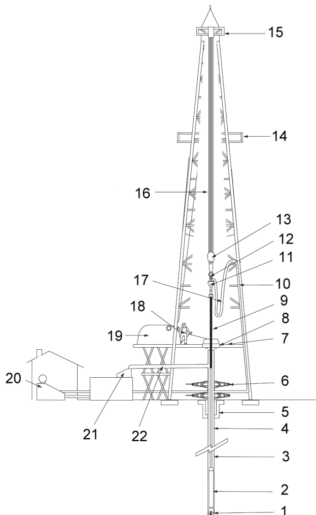
Рисунок 16.1 – Загальна схема бурової установки:
