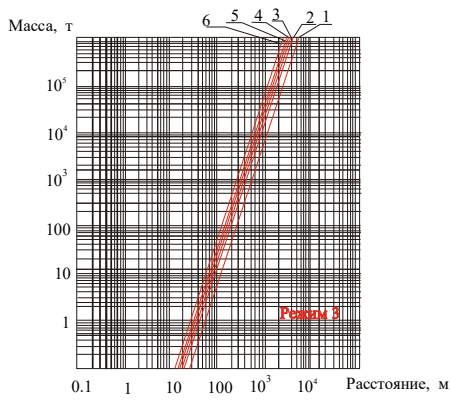
Рисунок 12.10 — Межі зон ураження людей при вибухах хмар ППС:
