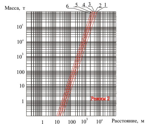
Рисунок 12.9 – Межі зон ураження людей при вибухах хмар ППС:
