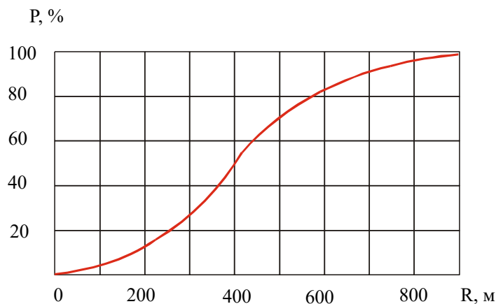
Рисунок 12.16 – Графік функції розподілу дальності розльоту осколків резервуару
