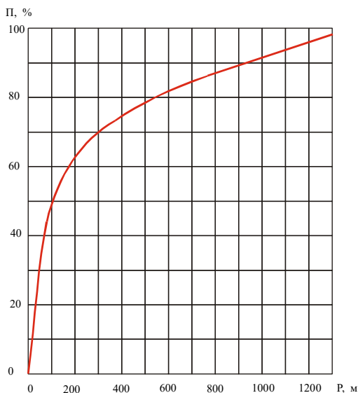
Рисунок 12.1 – Графік функції розподілу дрейфу хмари ППС
