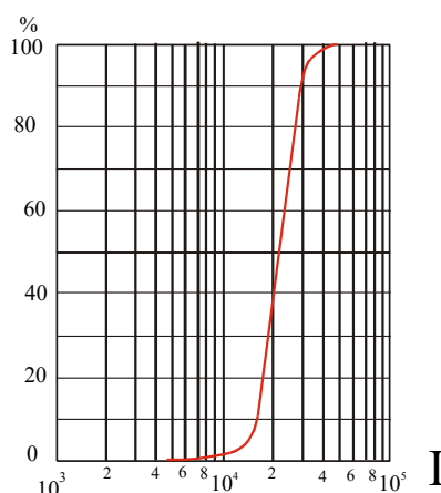
Рисунок 12.15 – Відсоток летальних випадків залежно від індексу дози теплового випромінювання I
