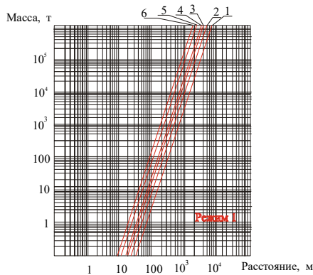
Рисунок 12.8 – Межі зон ураження людей при вибухах хмар ППС:
