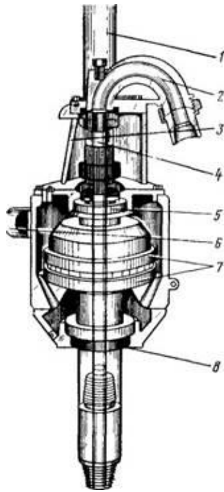
Рисунок 16.3 – Вертлюг:
