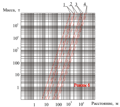
Рисунок 12.7 – Залежність ступеню руйнування будинку від маси палива й відстані:
