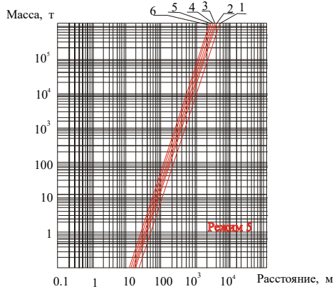
Рисунок 12.12 — Межі зон ураження людей при вибухах хмар ППС:
