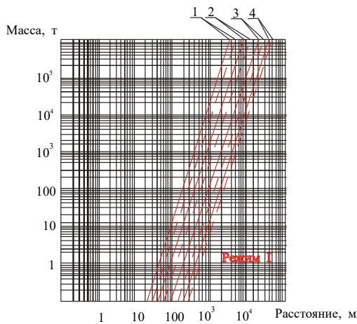
Рисунок 12.2 – Залежність ступеню руйнування будинку від маси палива й відстані:
