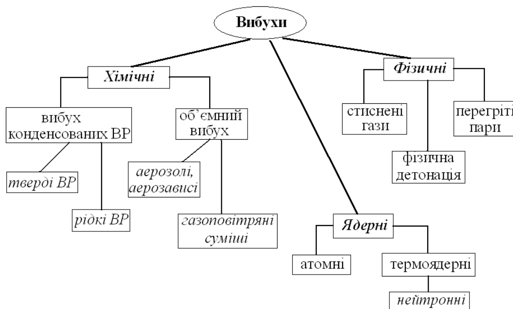
Рисунок 4.1 – Класифікація вибухів
