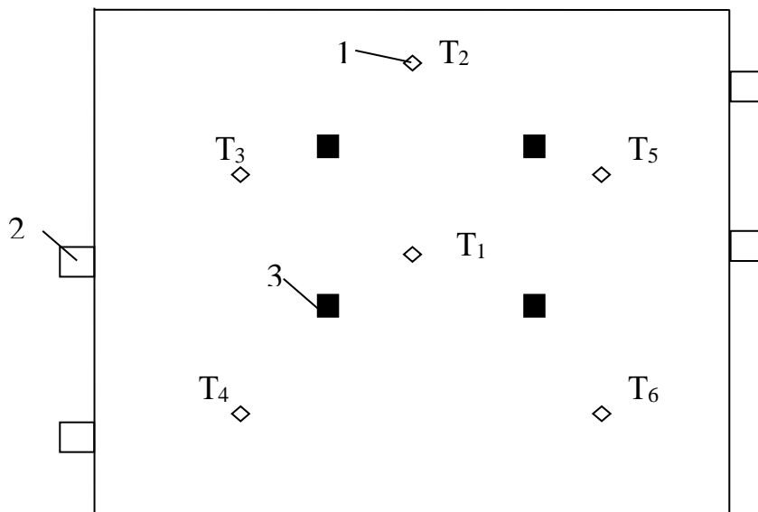
Рисунок 3.11 – Схема розміщення термопар для контролю температурного режиму в камері печі: T_1 – T_6 -термопари; 1 – розташування отворів для відводів продуктів горіння; 2 – пальник, 3 – отвір для виходу продуктів горіння
