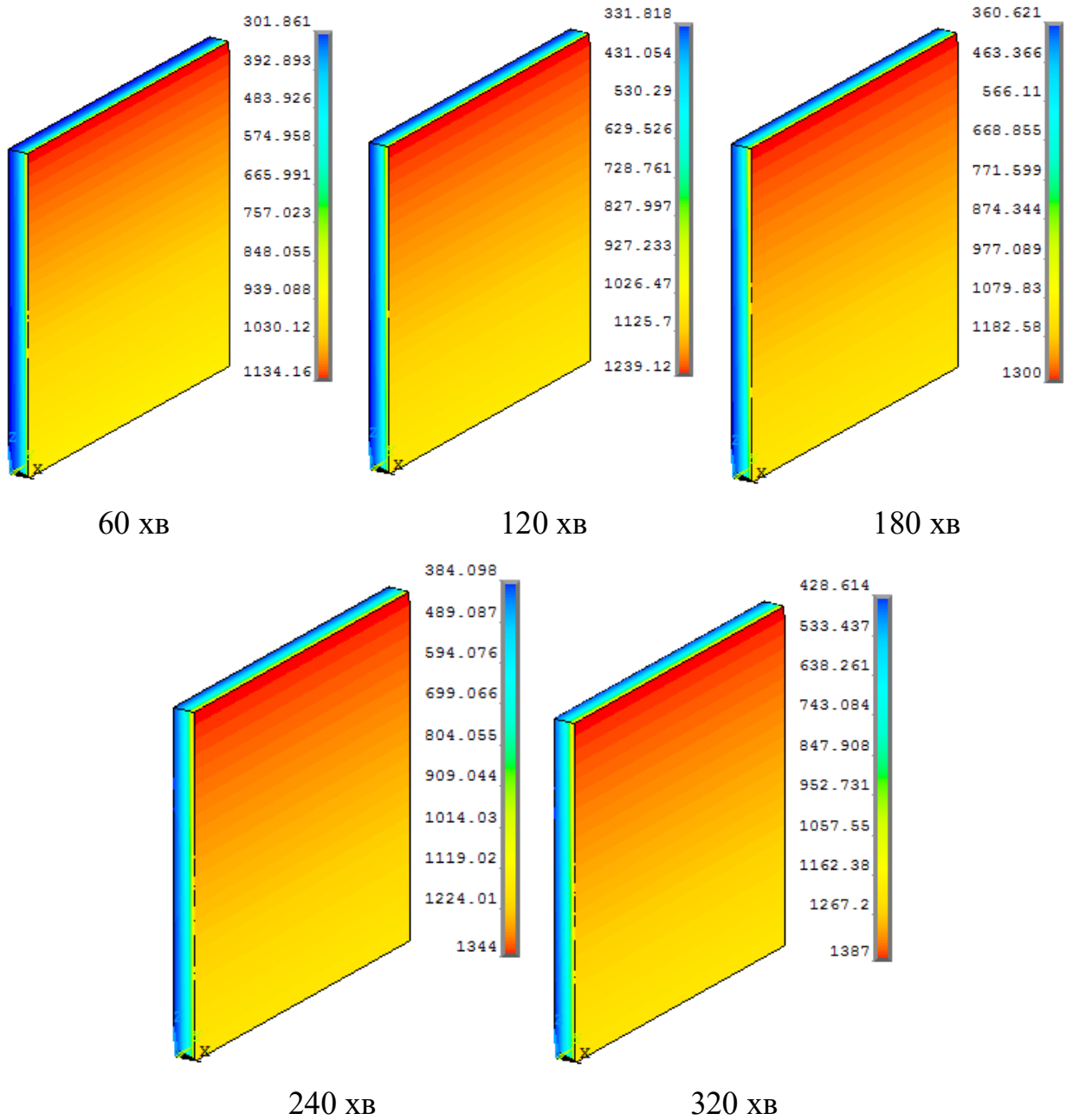
Рис. 5.7 – Температурні розподіли (К) у залізобетонній стіні, що були отримані у результаті теплотехнічного розрахунку, у різні моменти часу її вогневого випробування
