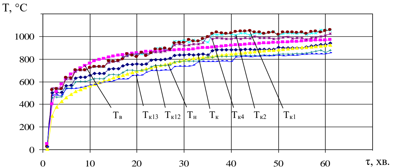
Рис. 2.11 – Графік зміни температури в печі Лаб. 2: T_{\max} – верхня межа випробувань; T_{\min} – нижня межа випробувань; T_{11} , T_{13} , T_{14} , T_{19} , T_{\Gamma} – показники всередині змодельованої термопарі в камері горизонтальної печі (рис. 2.7)
