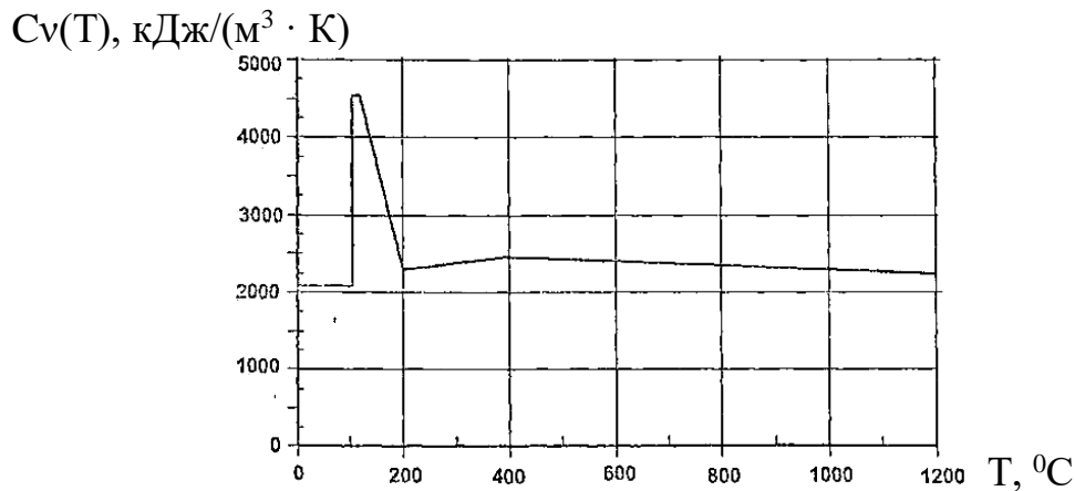
Рис. 1.8 – Залежність об'ємної теплоємності C_v(T) від температури для бетону густиною більше 2300 \text{ kg/m}^3 із вмістом масової вологості u=3\%
