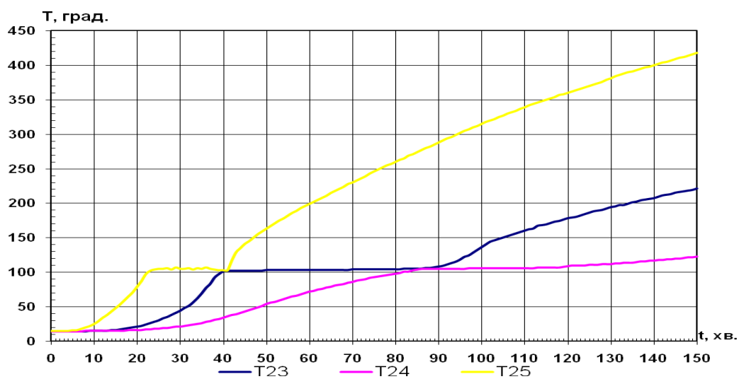
Рис. 3.6 – Залежності температури від часу на необігрівальній поверхні зразка
