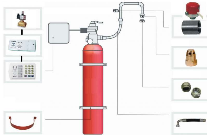
Рис. 1. Схема системи запобігання вибуху
