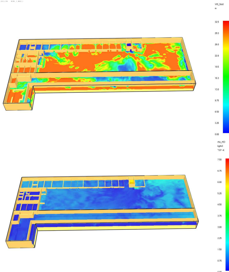
Рис. 1. Розподілення полів видимості та концентрацій HCl в приміщеннях.
