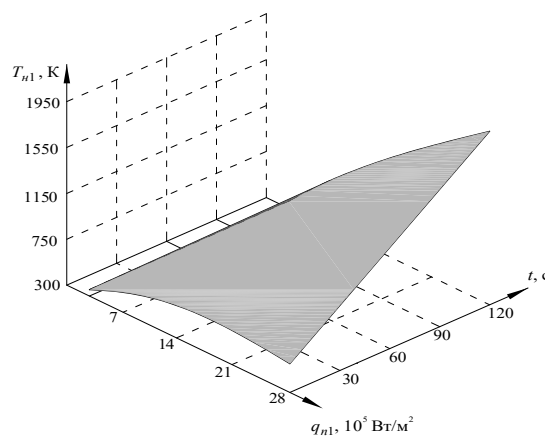
Рис. 2. Тривимірне зображення залежностей температури внутрішньої поверхні оболонки від величини зовнішнього теплового потоку та часу його дії ( T_0 = 300 К; r_2 - r_1 = 2 \cdot 10^{-3} м).
