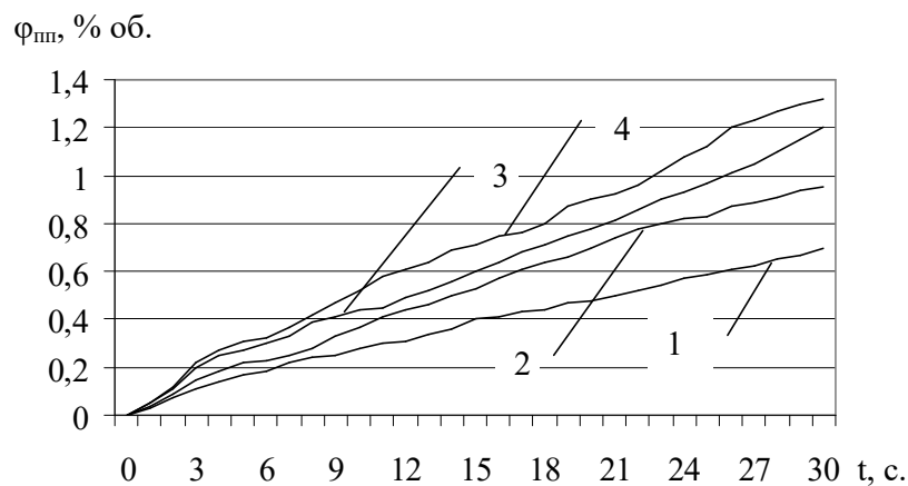
Рис. – Концентрація CO_2 в підмасочному просторі для лицьової частини різного типу: 1 – шолом-маска; 2 – шолом маска (переговорний пристрій); 3 – лицьова частина панорамного типу (MSA AUER); 4 – лицьова частина панорамного типу (ПМ-88)
