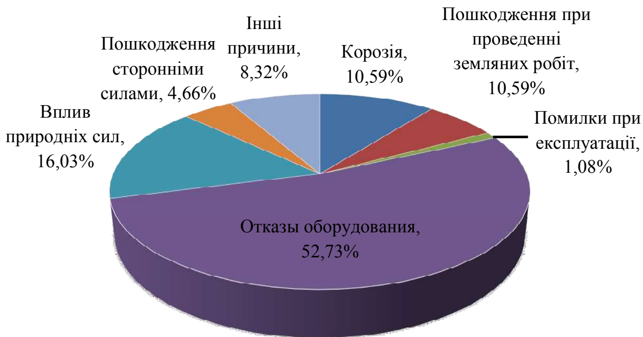
Рис. 2 – Причини відмов магістральних газопроводів
