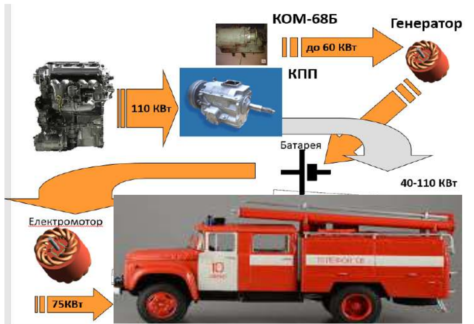
Рис. 3. – Загальна принципова схема трансмісії, що пропонується
