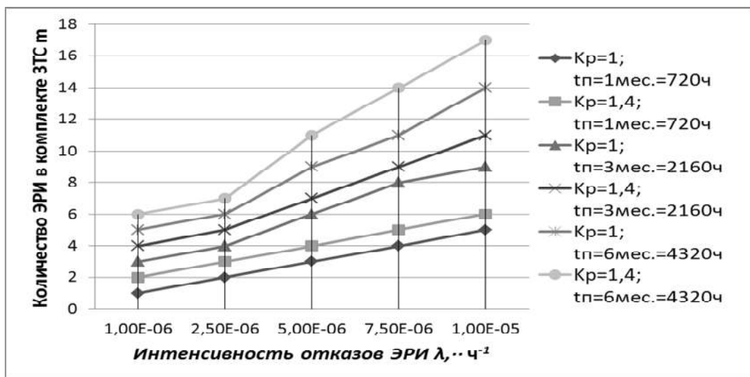
Рис. 1. График функции m = f(N, K_p, \lambda'_{\sigma}, t_n) , при K_p=1; 1,4; N=100; t_n=720ч; 2160ч; 4320ч, \lambda=10^{-6} - 10^{-5} ч^{-1}
