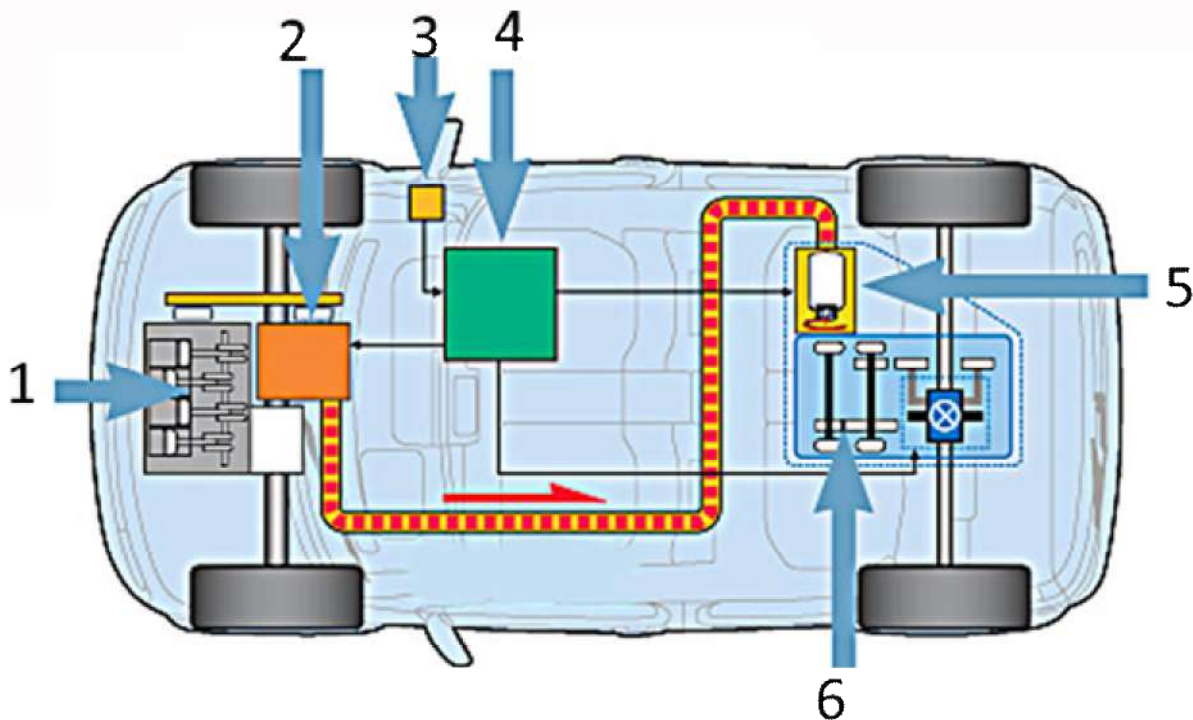
Рис. 2. – Принципова схеми трансмісії Nissan Tiida e-4WD: 1 - ДВЗ; 2 – вимикач; 3 - електрична машина – генератор; 4 – блок керування; 5 – електрична машина – електромотор; 6 – редуктор зі зчепленням.
