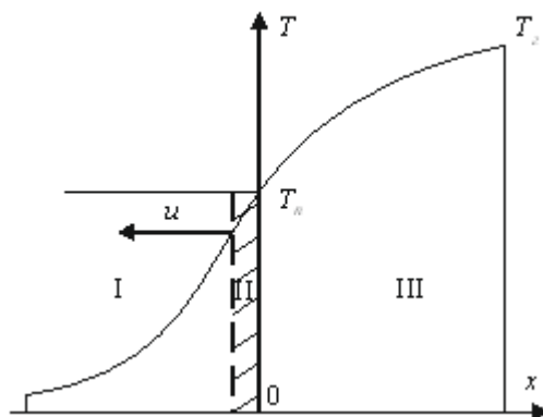
Рис. 1. – Схема розподілу температури поблизу поверхні горіння компонентів піротехнічної суміші
