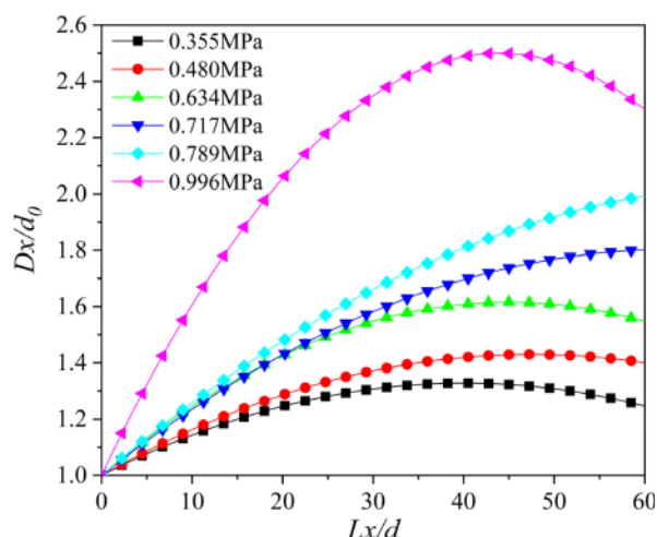
Рис. 2 – Залежність діаметра струменя та відстані від ствола при різних тисках [2]
