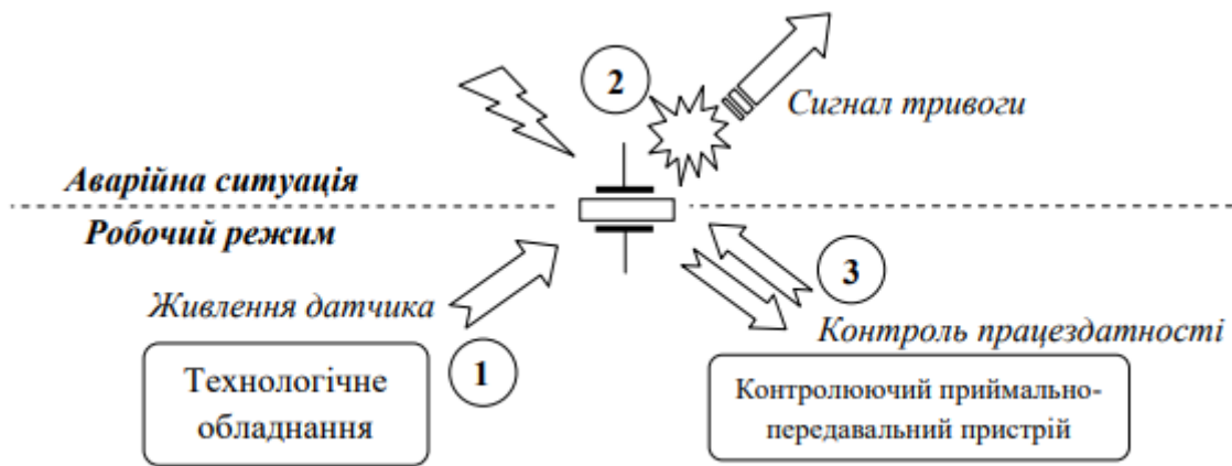
Рис. 1 – Принцип роботи п'єзотранспондера як датчика
