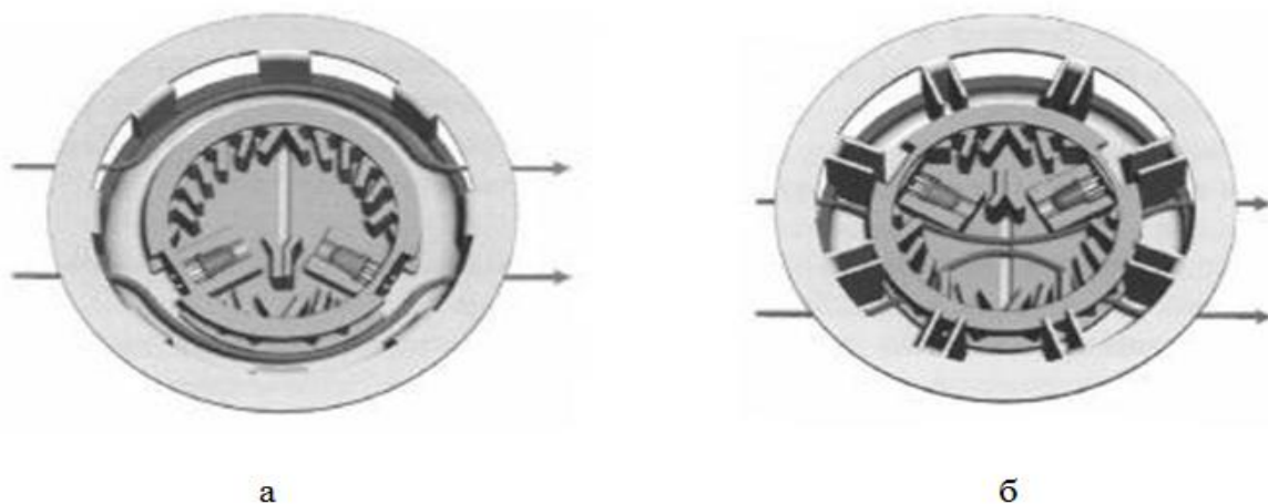
Рис. 2 – Схема вентиляції сповіщувача: а – некоректна; б – коректна
