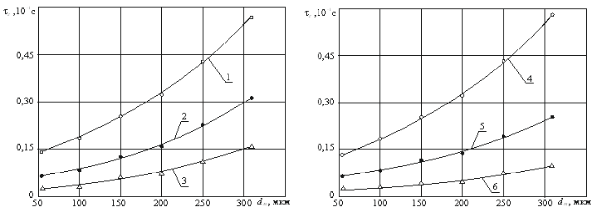
Рис. 1. – Вплив відносної концентрації кисню (а, P = 10^5 Па) та зовнішнього тиску (б, C_{O_2} = 0,4 ) на залежність часу згоряння частинки магнію у продуктах розкладання окиснювача від її розміру: 1 – C_{O_2} = 0,1 ; 2 – C_{O_2} = 0,4 ; 3 – C_{O_2} = 0,8 ; 4 – P = 10^5 Па; 5 – P = 10^6 Па; 6 – P = 3 \cdot 10^7 Па; \circ , \bullet , \Delta – експериментальні дані
