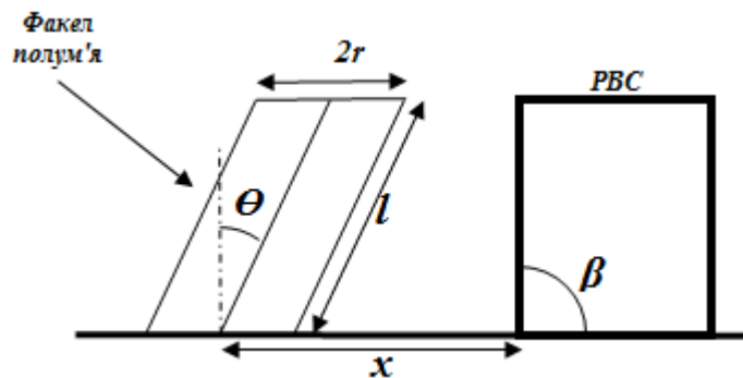
Рис. 1. – Схематичне зображення відхиленого факела полум'я
