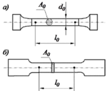
Рис. 1 – Зразки для випробування на розтяг
