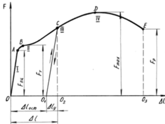
Рис. 2 – Діаграма розтягування зразка з маловуглецевої сталі
