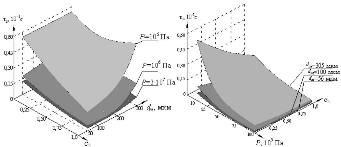
Рис. 2. – Тривимірне зображення залежностей часу згоряння частинки магнію у продуктах розкладання окиснювача: а) – від d_m та C_{O_2} ; б) – від C_{O_2} та P
