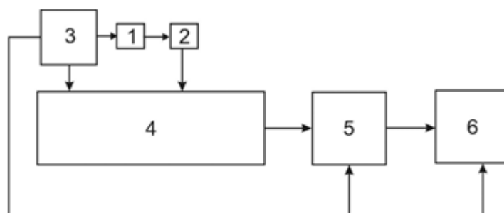
Рис. 1. – Функціональна схема пожежного сповіщувача на базі мобільного телефону: 1 – випромінювач інфрачервоного світла; 2 – фотоприймач. На фіг. 2 наведено функціональну схему індивідуального мобільного пристрою для виявлення диму, де: 3 – блок живлення; 4 – система обробки даних; 5 – пороговий пристрій; 6 – система оповіщення
