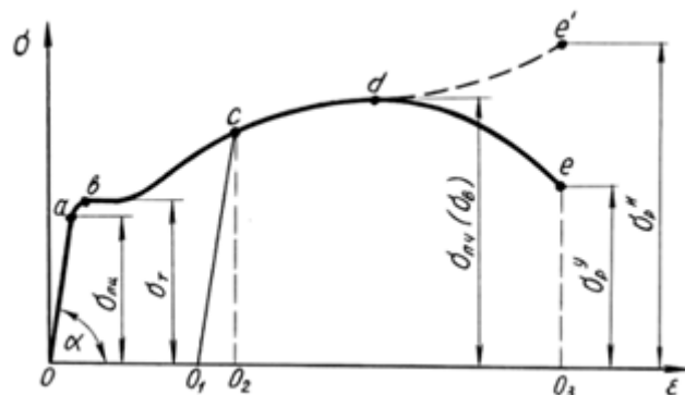
Рис. 3 – Умовна діаграма напруг при розтягуванні
