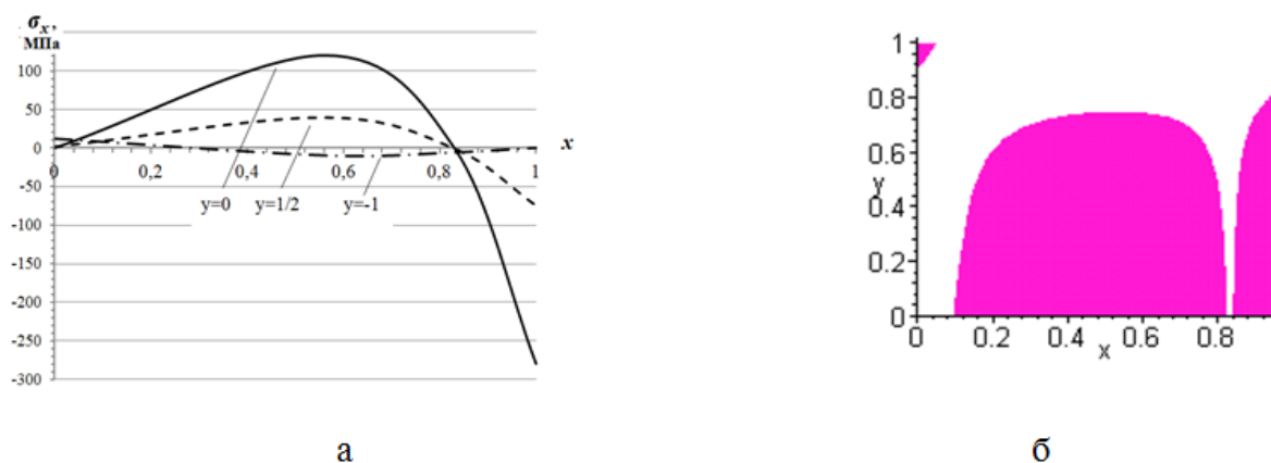
Рис. 1 – Розподіл нормальних напружень \sigma_x (а) та область тріщинуватості (б) (позначена темним кольором) в покрівлі при L \times B = 10 \times 10 \text{ м}^2 , H = 18,7 \text{ м}^2 , h = 0,4
