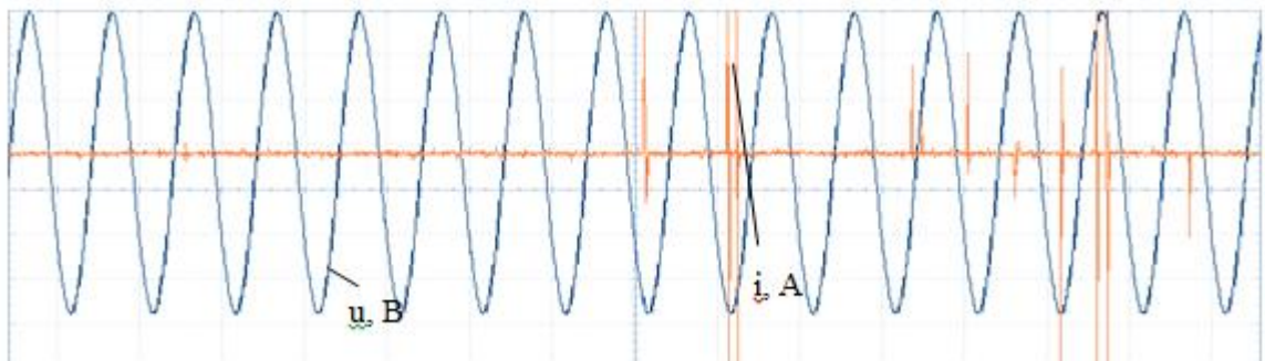
Рис. 1 – Осцилограма напруги і сили струму під час різання проводу марки СІП 2х16, диском діаметром 125 мм при частоті обертання в межах від 5500 до 5700 об/хв
