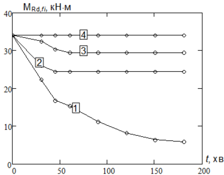
Рис. 2. – Графіки залежностей граничних пластичних моментів від значення часу тривалості пожежі відповідного стандартним класам вогнестійкості для залізобетонної плити товщиною 200 мм при різних температурних режимах пожежі: 1 – стандартний температурний режим; 2 – температурний режим, розрахований при коефіцієнті прорізів O = 0.0045 \text{ м}^{0.5} та щільності пожежного навантаження q_{t,m} = 1200 \text{ МДж/м}^2 ; 3 – температурний режим, розрахований при коефіцієнті прорізів O = 0.0045 \text{ м}^{0.5} та щільності пожежного навантаження q_{t,m} = 850 \text{ МДж/м}^2 ; 4 – температурний режим, розрахований при коефіцієнті прорізів O = 0.0045 \text{ м}^{0.5} та щільності пожежного навантаження q_{t,m} = 500 \text{ МДж/м}^2
