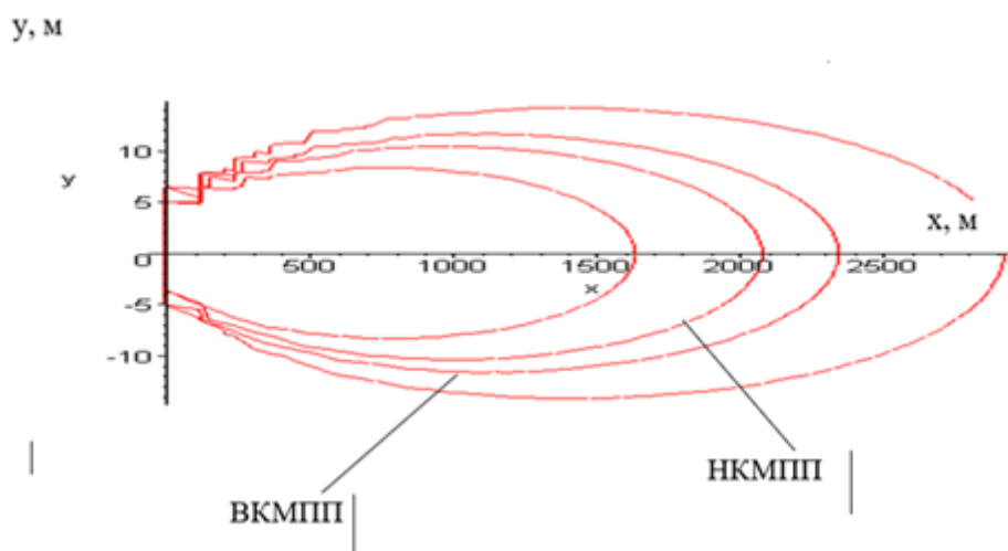
Рис. 1. – Результати розрахунків НКМПП і ВКМПП
