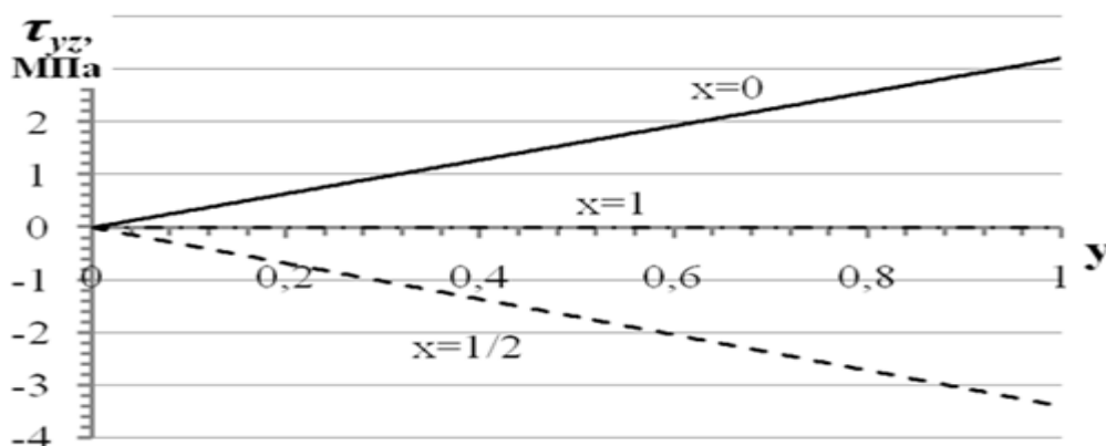
Рис. 2 – Розподіл поперечних дотичних напружень \tau_{yz} в покрівлі без врахування тріщинуватості при L \times B = 10 \times 10 \text{ м}^2 , H = 18,7 \text{ м}^2 , h = 0,4
