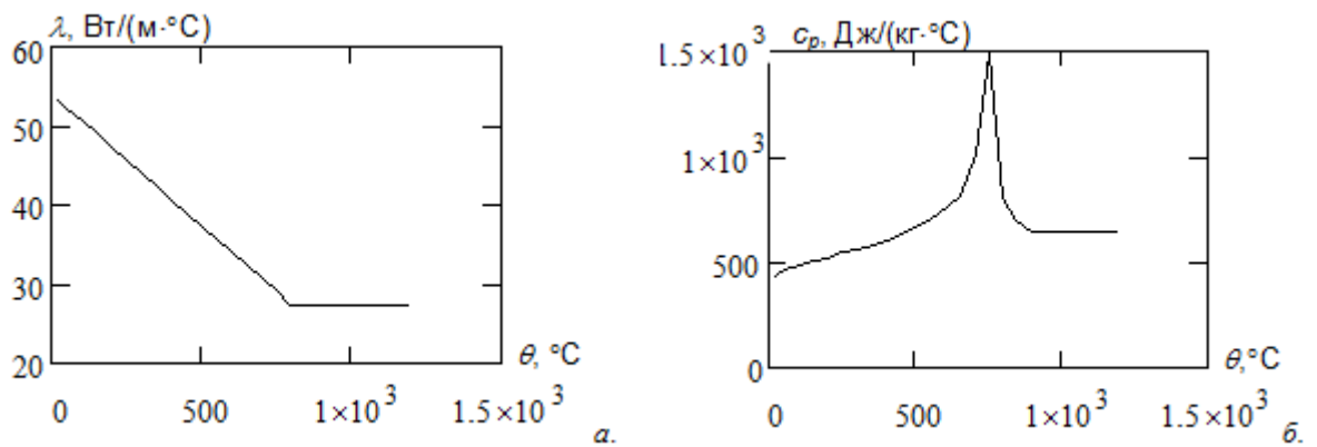
Рис. 2. – Теплофізичні характеристики сталі: коефіцієнт теплопровідності (а); питома теплоємність (б)
