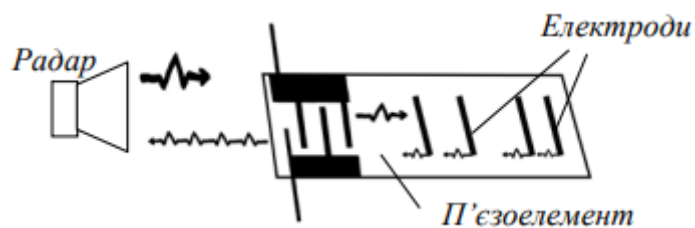
Рис. 2 – П'єзоперетворювач як транспондер
