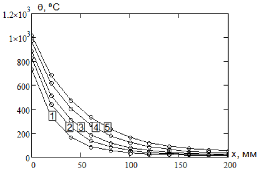
Рис. 2. – Розподіли температури по перерізу залізобетонної плити для стандартного температурного режиму пожежі у час температурного впливу пожежі відповідного стандартного класу вогнестійкості: 1 – 30 хв., 2 – 45 хв., 3 – 60 хв., 4 – 90 хв., 4 – 120 хв.
