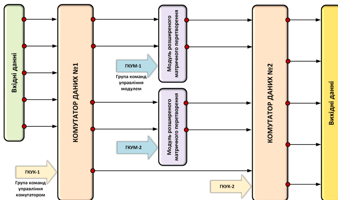
Рис. 1. – Модель процесу реалізації операцій розширеного матричного криптографічного перетворення
