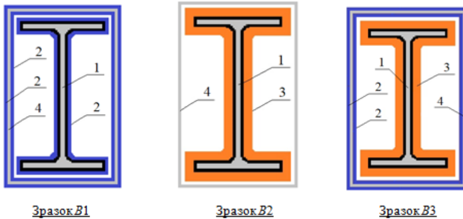
Рис. 1. – Конструкція експериментальних зразків групи А
