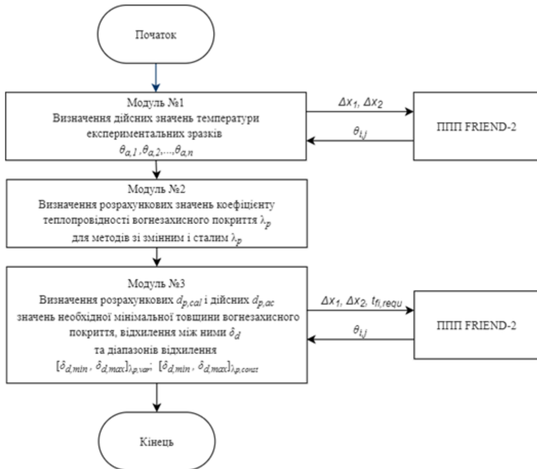
Рис. 1. – Блок схема алгоритму автоматизованої реалізації процедури валідації методів розрахунку характеристики вогнезахисної здатності покриттів
