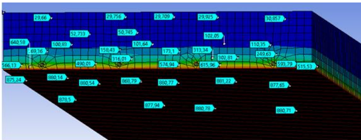
Рис. 4 – Поширення температури в результаті теплового впливу стандартного температурного режиму пожежі
