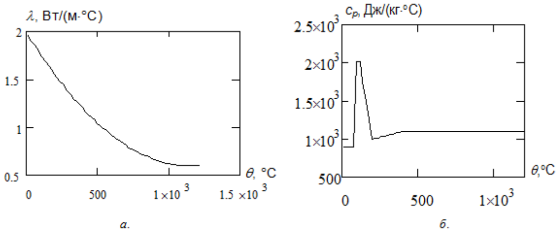
Рис. 1. – Теплофізичні характеристики важкого бетону на гранітному заповнювачі: а – коефіцієнт теплопровідності; б – питома теплоємність
