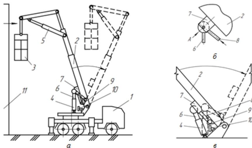
Рис. 2 – Підйомник з автоматичним відходом обладнання під час руйнування об'єкта: а – загальний вид; в – фіксатор гідроциліндра керування стрілою; б – механізм керування
