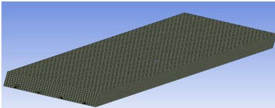
Рис. 3 – Сіткова модель залізобетонної плити
