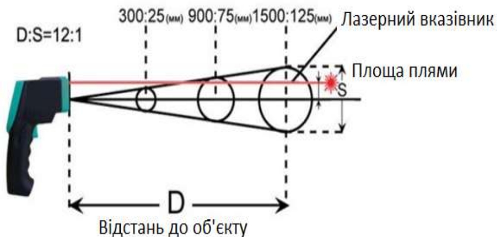
Рисунок 1 – Схема роботи пірометра
