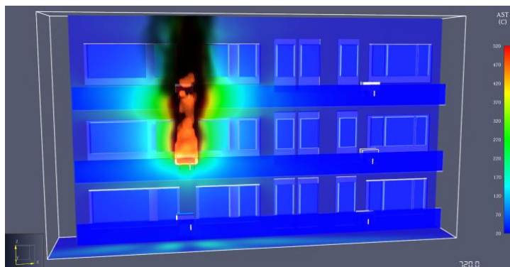
Рис. 1 Візуалізація пожежі зовнішнього блоку кондиціонера та температурного розподілу по фасаді будівлі
