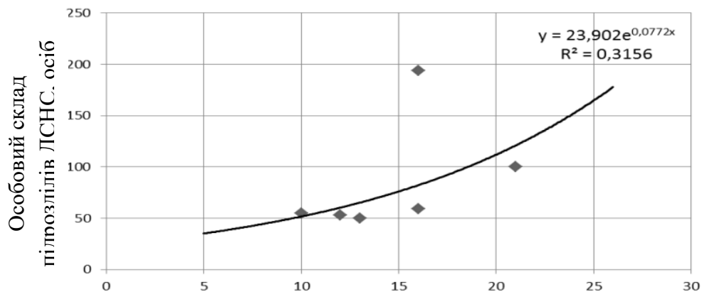
Рис 1. Залежність кількості особового складу, залученого до гасіння великих пожеж на полігонах ТПВ від кількості пожежних автомобілів
