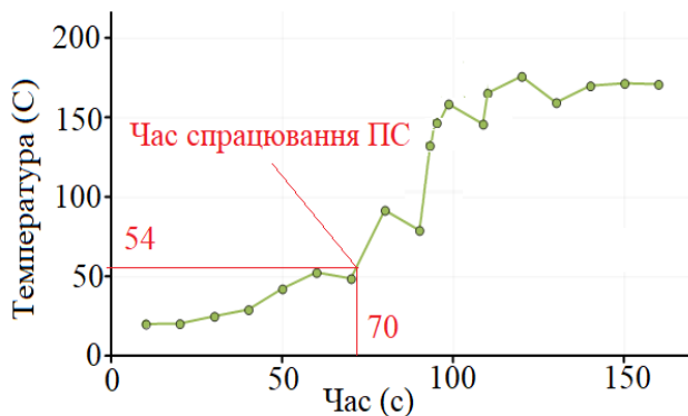
Рис. 3. Час спрацювання сповіщувача
