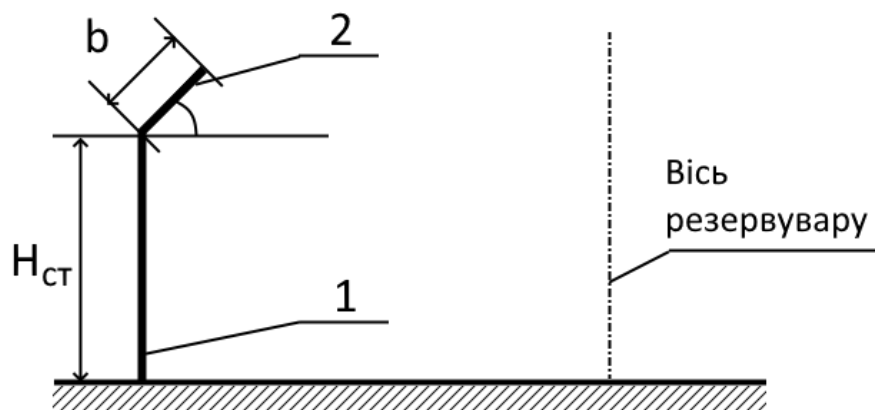
Рис. 1. Схема захисної стінки: 1 – захисна стінка; 2 – хвилевідбивний козирок
