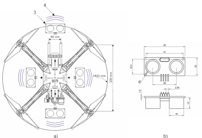
Рис. 1. а) – схема розміщення акустичних датчиків на корпусі мікродрону (вид згори, 1 – акустичний датчик, 2 – напрямок дії акустичних хвиль); б) – схема будови акустичного датчика
