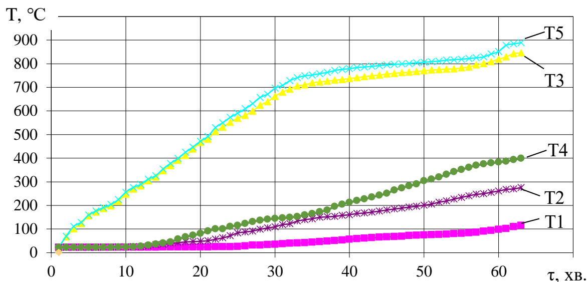
Рисунок 3 – Результати вимірювання температури досліджуваного зразка: T1-T5 – показання термопар (рис. 2.)
