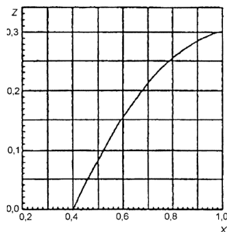
Рисунок 1 – Графік значення коефіцієнта Z участі парів легкозаймистих рідин у вибуху
