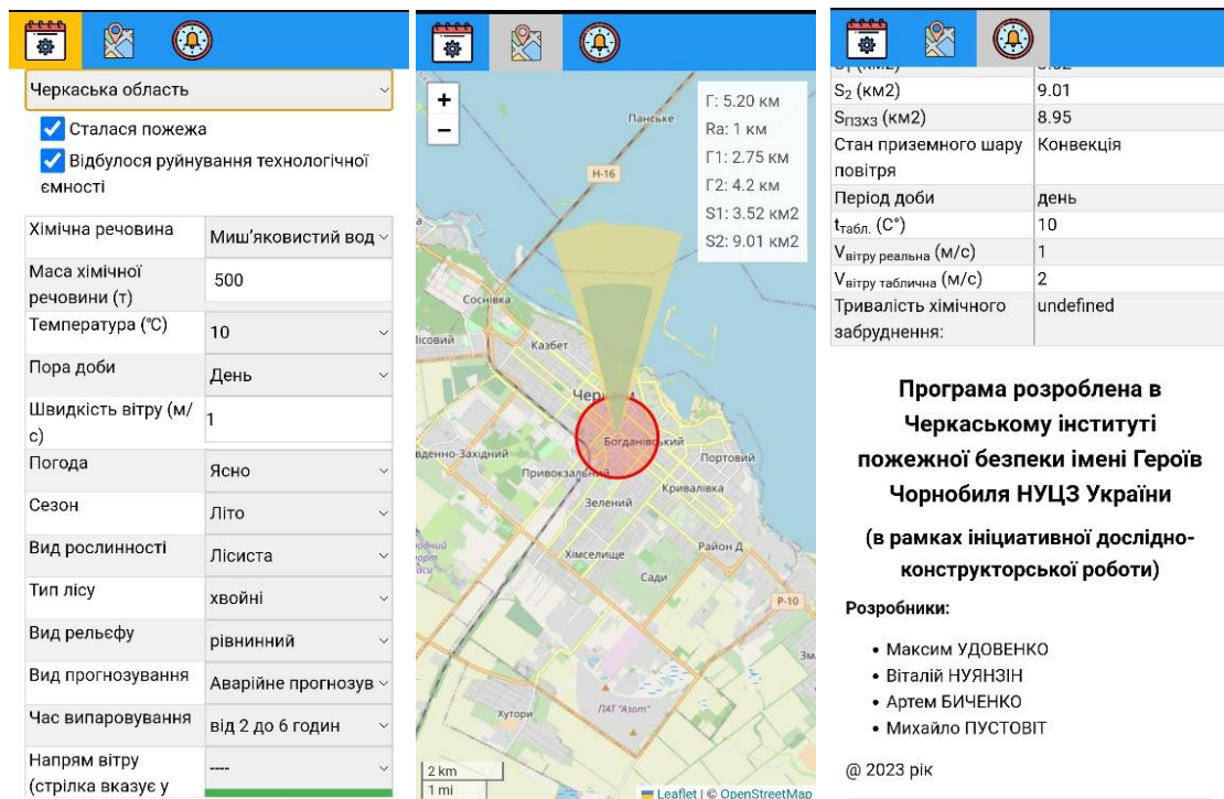
Рис. 2. Мобільний android-додаток для проведення оцінки обстановки при аваріях на хімічно небезпечних об'єктах і транспорті
