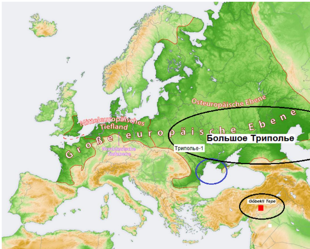
Рис. 5. Локалізація пенепленів на теренах Європи (замкнені чорні і червоні лінії, а синім вказано місце перебування пращурів в дельтах рік, що впадали в прісну Понтиду)
