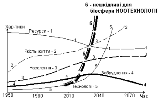
Рис. 2. Удосконалена введенням екоідеальних ноотехнологій «текстуальна» модель №13 з книги «Межі зростання», яка розпочала ставати реальністю з 2000 року
