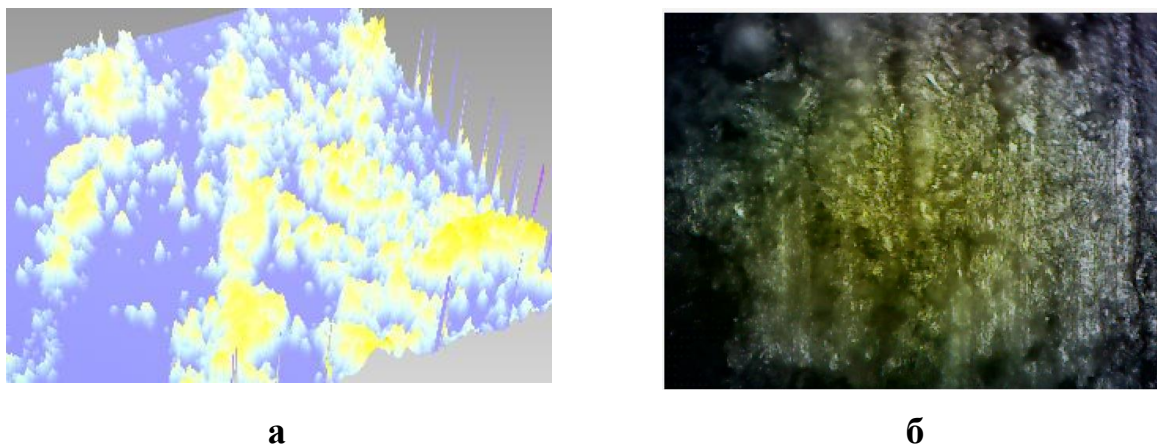
Рис. 4. Поверхня валу після струменево-абразивної обробки: а - 3-D топографія поверхні; б - макрошліф поверхні
