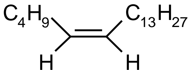
Рис. 2. Z-5-нонадецен
