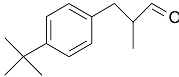
Рис. 3. Ліліаль
