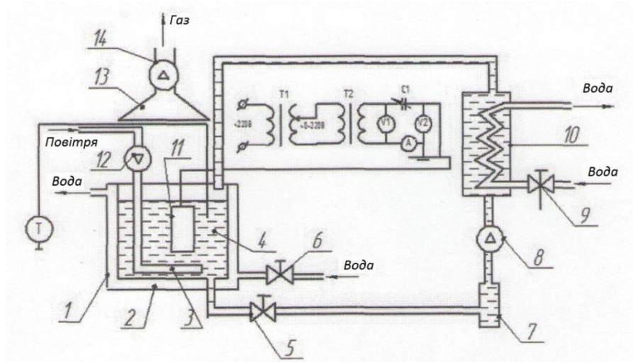
Рис. 3. Функціональна схема установки пароплазмового нанесення: 1-гальванічна ванна; 2-рубашка водяного охолодження; 3-барботер; 4-електроліт; 5,6,9-запорна арматура; 7-фільтр; 8-водяний насос; 10-бак з теплообмінником; 11-деталь; 12-повітряний компресор; 13-витяжний зонт; 14-витяжний вентилятор
