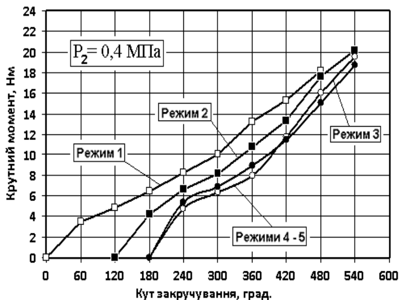
Рисунок 1 – Діаграми нагрузок испытательного фрагмента пожарного рукава при кручении (давление в рукаве P_1 = 0,4 МПа)
