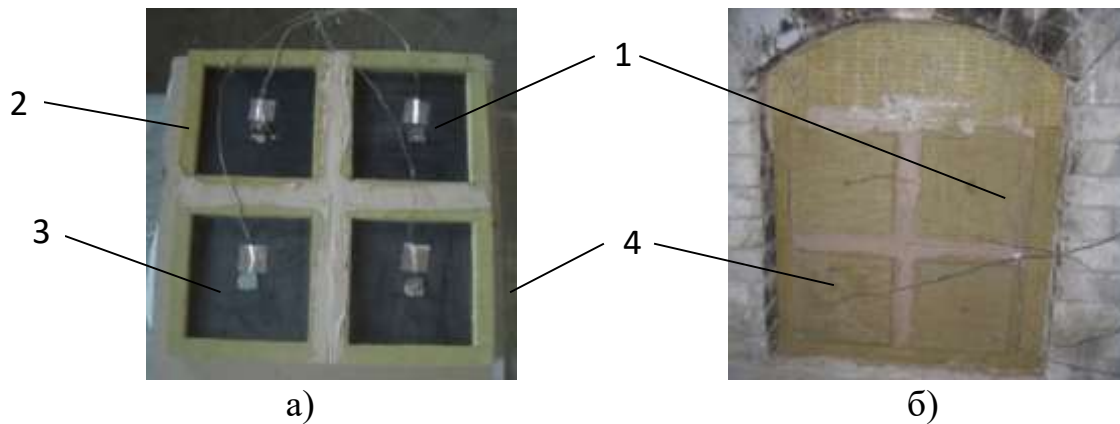
Рисунок 1 – Зразки (а): 1-термопара типу ТХА, 2-опорна конструкція для зразків, 3-сталева пластина з нанесеним вогнезахисним покриттям, 4-теплоізоляційна плита Rockwool і вертикальна випробувальна піч (б).
