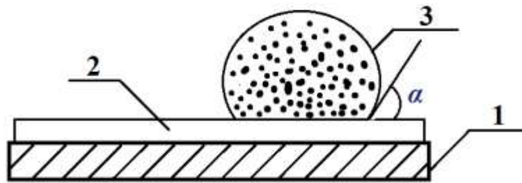
Рисунок 1 – Схема заміру поверхневого натягу на поверхні сажі та золи. 1) підложка; 2) шар аерозольних продуктів горіння (сажа, зола); 3) крапля контрольної рідини (вода або водний розчин ПАР).
