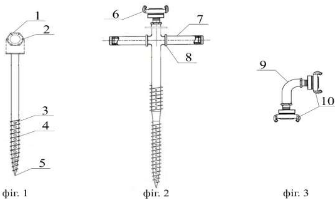
Рисунок 1 – Спеціальний пожежний ствол для гасіння підземних пожеж:
