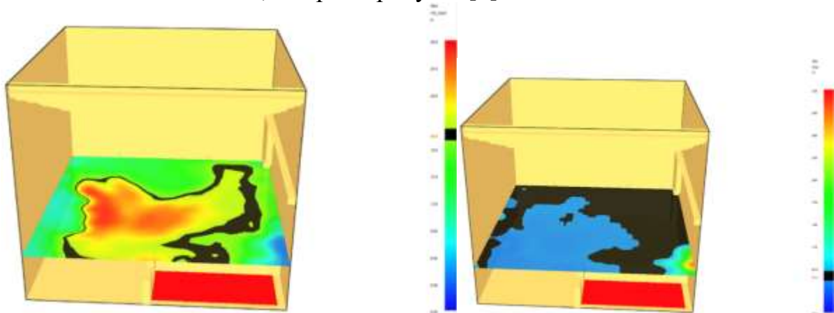
Рисунок 2 – Розподілення полів видимості (а) та температурних полів (б) в приміщенні
