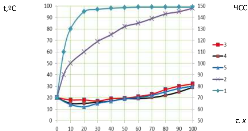
Рисунок 1 – Результати експериментальних досліджень динаміки температури на зовнішній поверхні (1), у просторі під одягом у ділянці основної частини тіла (3), кистей рук (4), стоп ніг (5) і ЧСС (2) у костюмі з системою охолодження
