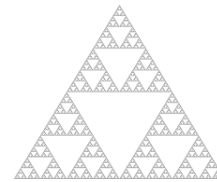
Рис. 3 Трикутник Серпінського
