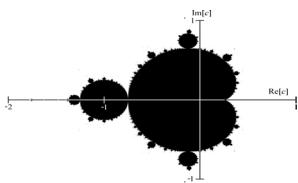
Рис. 1 Множина Мандельброта
