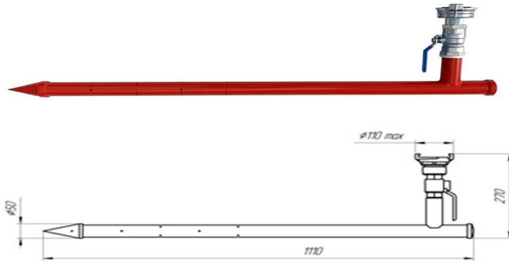
Рис. 1. Ствол-пробійник пожежний ручний СППР-50
