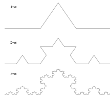
Рис. 2 Крива Коха
