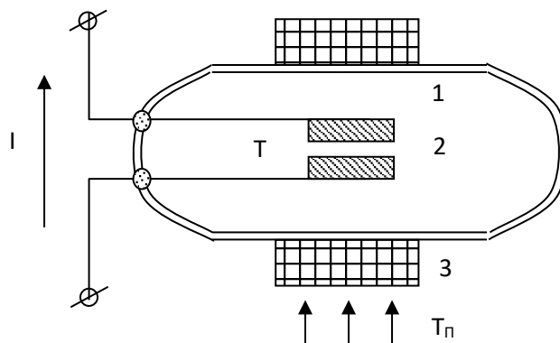
Рисунок 1 – Розрахункова схема теплового СП: 1 – геркон; 2 – феритові контакти; 3 – кільцевий постійний магніт
