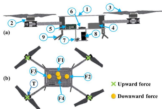
Рисунок 1 – (a), компоненти квадрокоптера, (1) корпус квадрокоптера, (2) двигуни BLDC, (3) гвинти, (4) акумулятор, (5) USRP E312, (6) Pixhawk контролер польоту, (7) ширококутова камера, (8) приймач FSO та (9) антени
