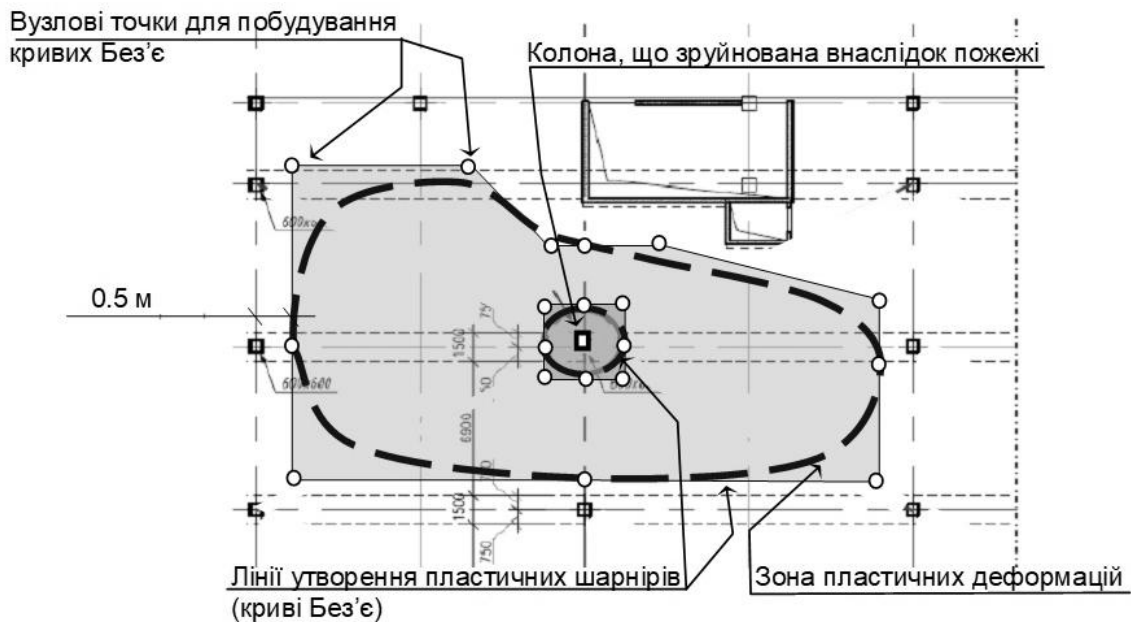
Рисунок 2 – Відтворення ліній утворення пластичних шарнірів за допомогою кривих Без'є.
