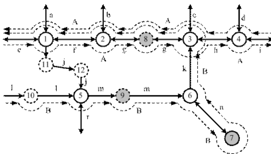
Рис. 2. Приклад даних моделі «транспортна мережа»: 1-7 – вузли; 8-12 – проміжні точки; 7-9 – зупинки; a-n – дуги; A-V – маршрути громадського транспорту
