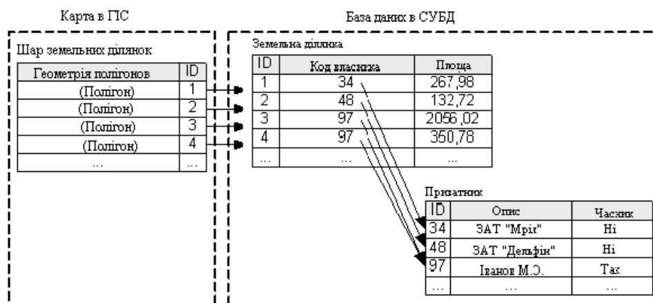
Рис. 5 Георефлексна база даних: а – впорядкований список просторових об'єктів в шарі карти; б – пов'язані з ними записи в базі даних
