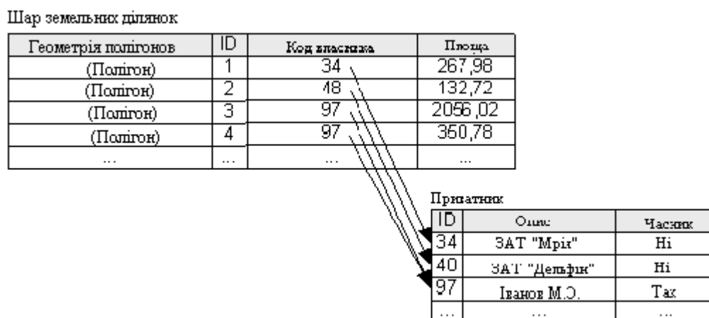
Рис. 6 З'єднання таблиць георефлексної бази даних
