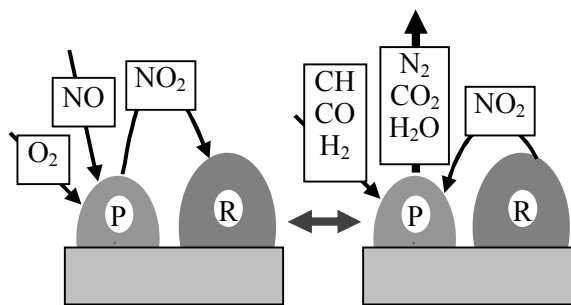
Рис. 4. Схема работы катализатора накопительного типа: слева – в цилиндрах двигателя сгорает бедная горючая смесь, справа – смесь стехиометрического или богатого состава
