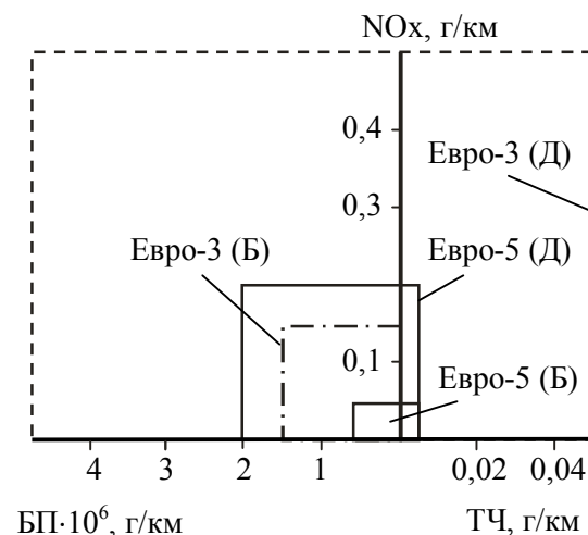
Рис. 2. Эволюция международных норм на уровни выбросов вредных веществ (NOx, ТЧ, а также БП) с ОГ дизелей (Д) и бензиновых (Б) двигателей, определяющих экоканцерогенную опасность легковых автомобилей
