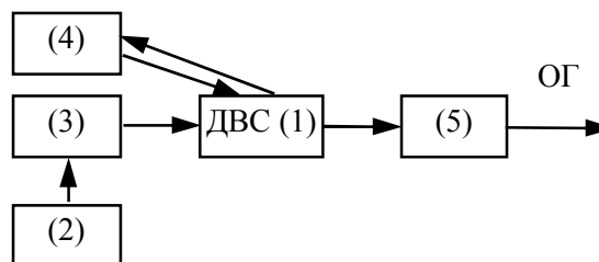
Рис. 5. Схема современной системы управления и регулирования энергоустановки автомобиля
