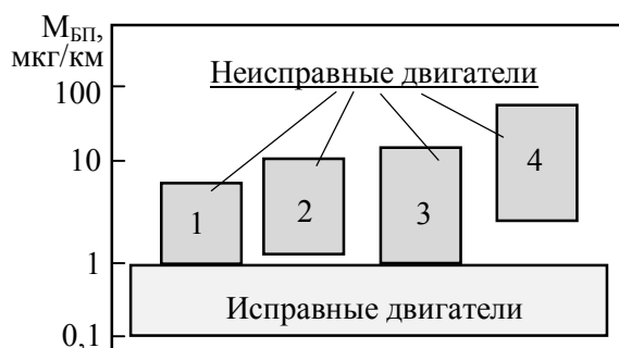
Рис. 1. Уровни выброса бенз(а)пирена с ОГ автомобилей при различных неисправностях бензиновых двигателей: 1 – нарушение регулировки холостого хода, 2 – угар масла, 3 – неисправности системы питания, 4 – неисправности системы зажигания
