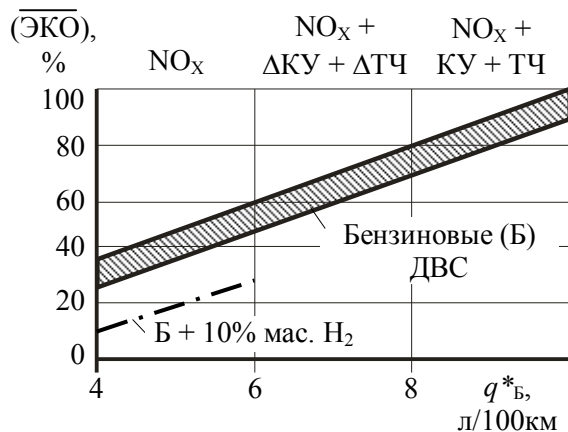
Рис. 3. Относительная экотоксичность легковых автомобилей с ДВС в зависимости от их эксплуатационной экономичности: q^*_Б – приведенный расход бензина по городскому ездовому циклу
