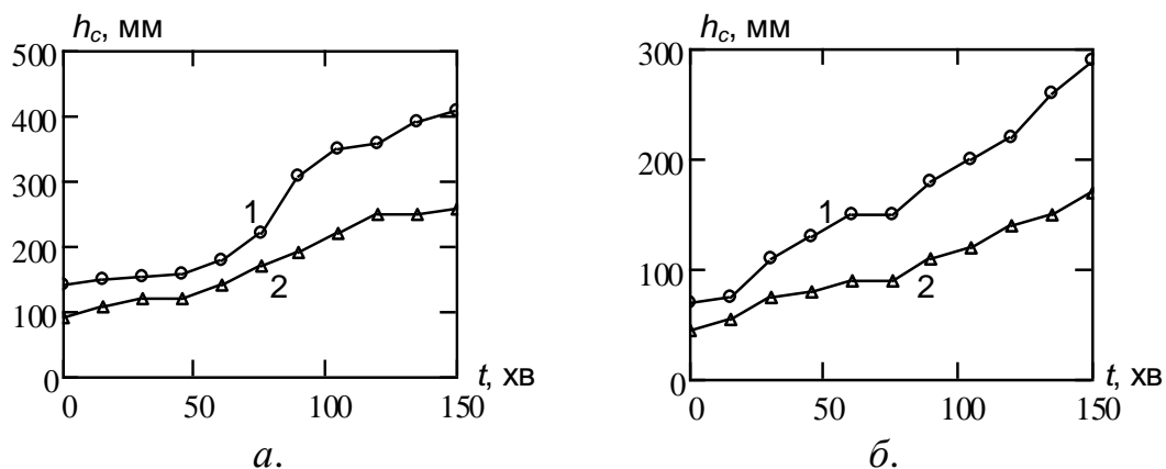
Рис. 4.17. Залежність середньої висоти нормальних тріщин (а) та торцевих тріщин (б): 1 - сталезалізобетонних плит пешого типу; 2 – сталезалізобетонних плит другого типу.
