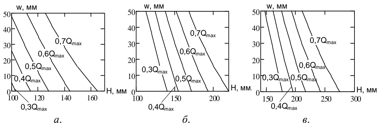
Рис. 5.2. Залежності захисного шару бетону від висоти двотаврового сталевого елемента сталезалізобетонної плити для забезпечення межі вогнестійкості: а – R 120; б - R 180; в - R 240
