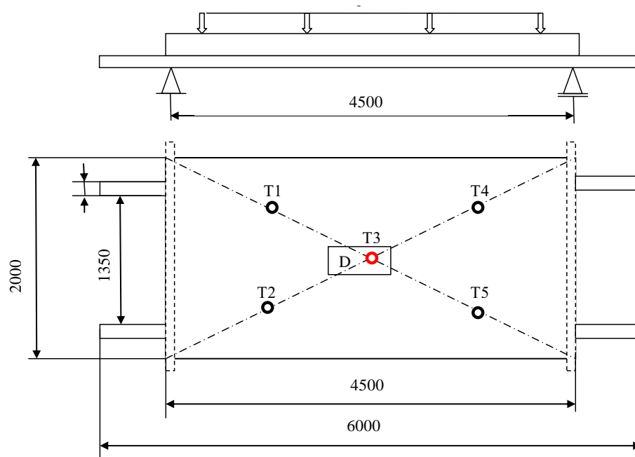
Рис. 3.9. Схема розташування термопар у перерізі сталезалізобетонної плити-зразку для випробувань.
