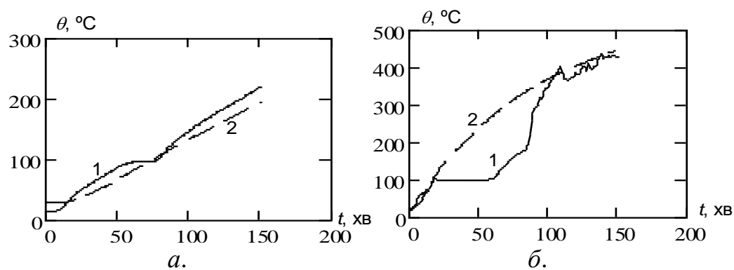
Рис. 4.19. Експериментальні (1) та розрахункові (2) показники температури у середині двотавра при випробуванні сталезалізобетонних плит: а – першого типу; б – другого типу.
