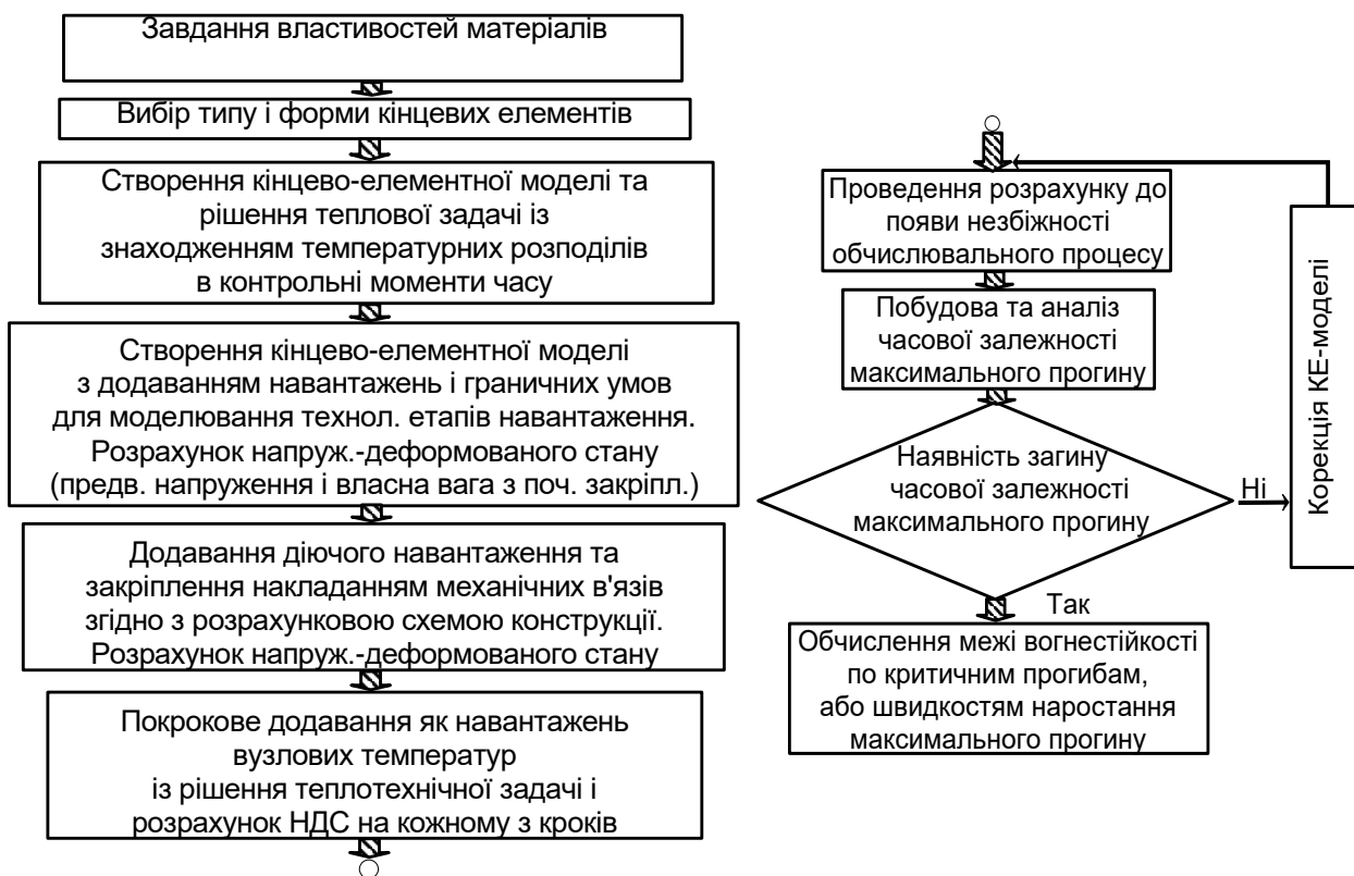
Рис. 2.18. Структурна схема розрахункових процедур щодо визначення параметрів напружено-деформованого стану сталевих залізобетонних плит.
