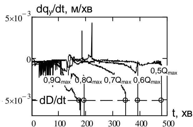
Рис. 2.30. Графіки швидкості наростання найбільшого прогину сталезалізобетонної плити у залежності від часу її експонування в умовах пожежі із стандартним температурним режимом для різних умов навантаження.
