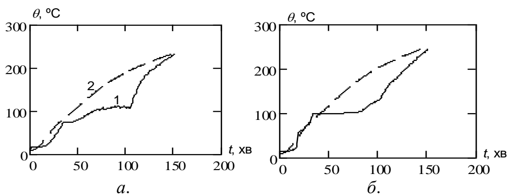
Рис. 4.18. Експериментальні (1) та розрахункові (2) показники температури у середньому арматурному стержні при випробуванні сталезалізобетонних плит: а – першого типу; б – другого типу.
