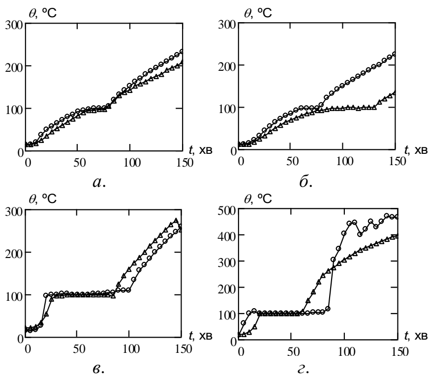
Рис. 4.7. Показники термопар посередині стінки сталевого двотаврового елементу сталезалізобетонних плит: а – першого зразка першого типу плити; б – другого зразка першого типу плити; в – першого зразка другого типу плити; г – другого зразка другого типу плити;
