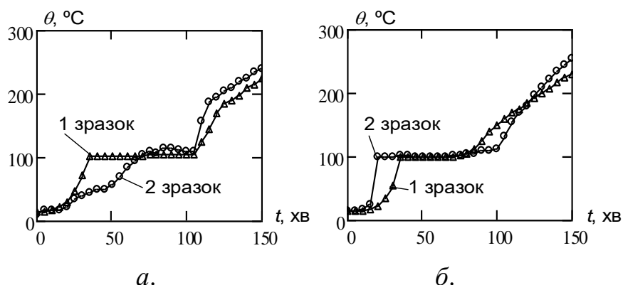
Рис. 4.8. Показники термопар у середньому арматурному стержні посередині сталезалізобетонних плит: а – зразків першого типу плити; б – зразків другого типу плити.
