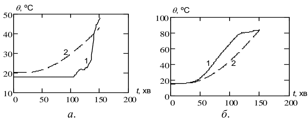
Рис. 4.20. Експериментальні (1) та розрахункові (2) показники температури на необігрівній поверхні при випробуванні сталезалізобетонних плит: a – першого типу; б – другого типу.
