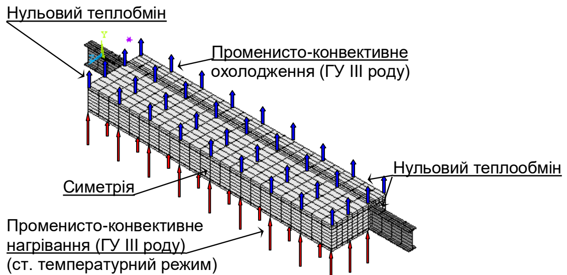
Рис. 2.7. Схема прикладання граничних умов до кінцево-елементної схеми сталезалізобетонної плити
