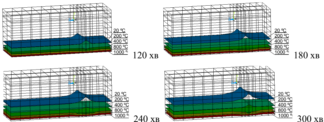
Рис. 2.8. Результати вирішення теплотехнічної задачі: температурні розподілення у перерізі сталезалізобетонної плити у різні моменти часу
