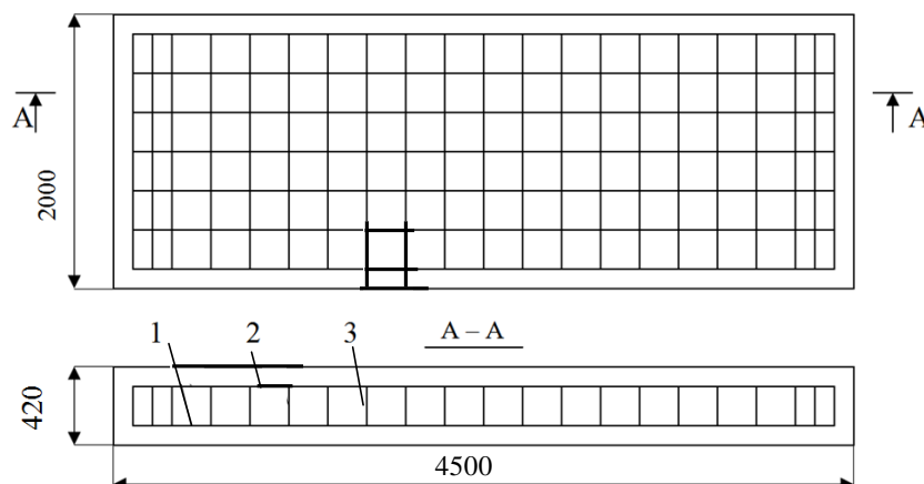
Рис. 3.7. Схема досліджуваної стале залізобетонної плит: 1 – арматура d = 12 мм А500С; 2 – арматура d = 10 мм А240С; 3 – арматура d = 8 мм А240С.
