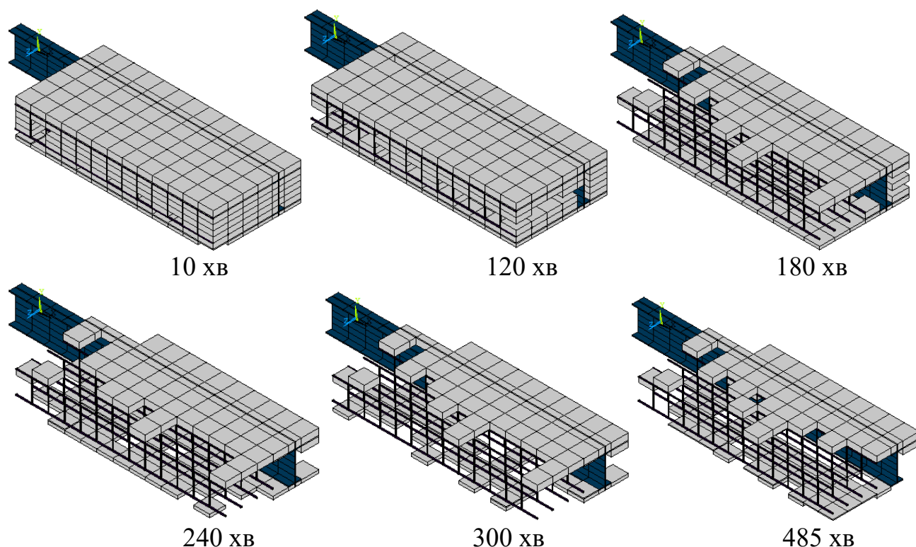
Рис. 2.26. Розподіли роздроблених елементів у шарах бетону сталезалізобетонної плити в умовах пожежі із стандартним температурним режимом у різні моменти часу.
