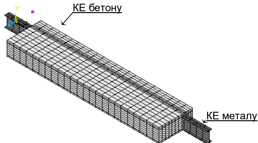
Рис. 2.6. Кінцево-елементна схема сталезалізобетонної плити
