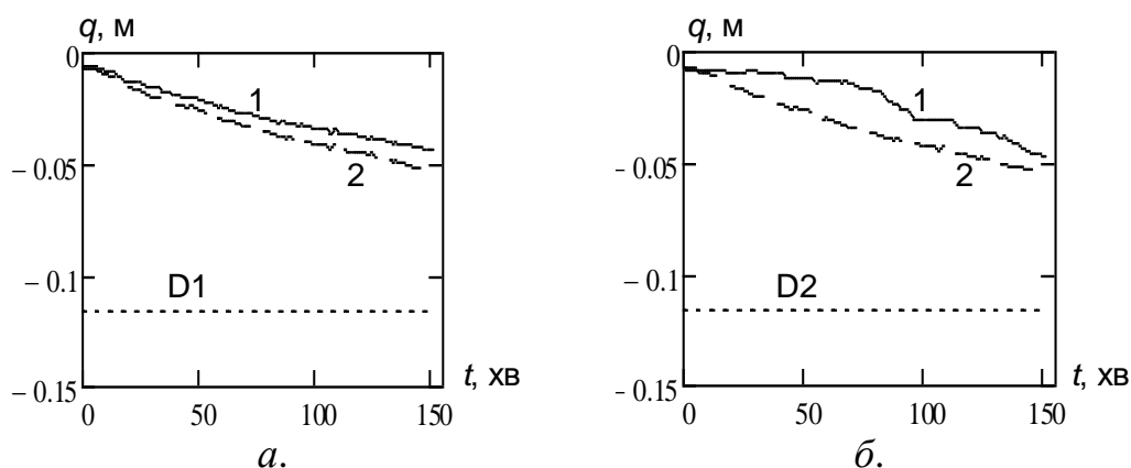
Рис. 4.21. Залежність середнього експериментального (1) та розрахункового (2) значень максимального прогину сталезалізобетонних плит із відхиленнями: a – зразків першого типу плити; б – зразків другого типу плити;
