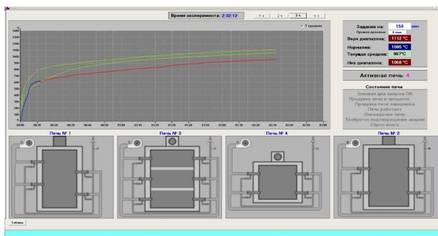
Рис. 3.4. Интерфейс программного обеспечения системы контролю температур.
