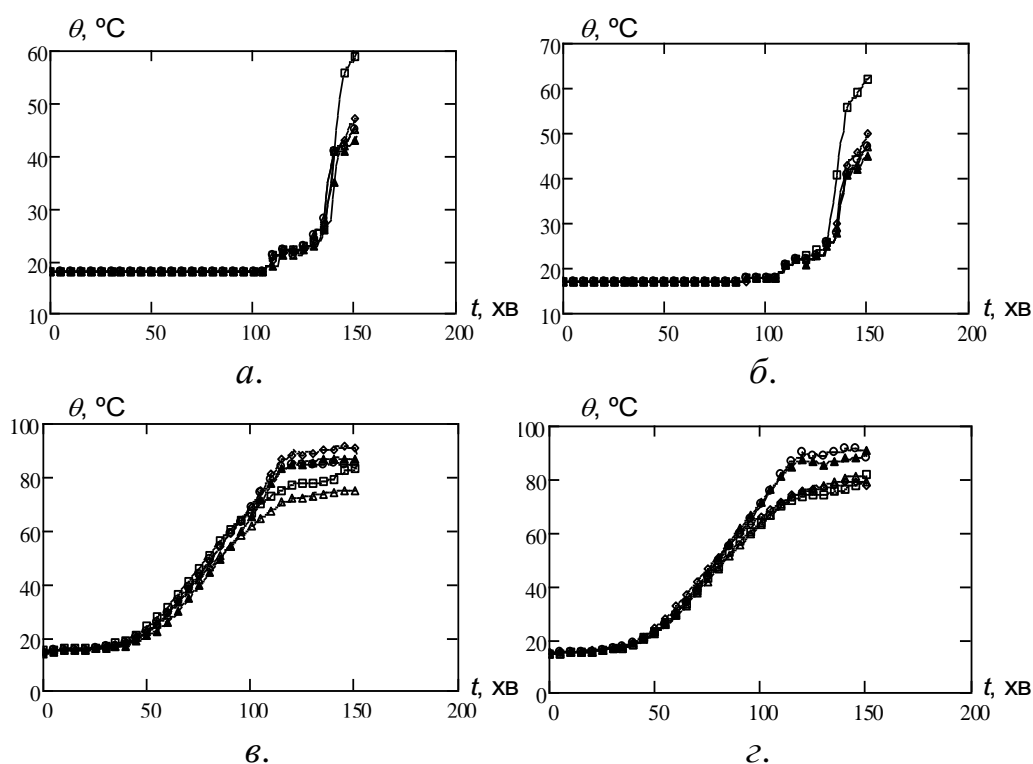
Рис. 4.11. Показники термомпар на необігрівній поверхні сталезалізобетонних плит першого типу зразків №1 ( а ) та №2 ( б ), сталезалізобетонних плит другого типу зразків №1 ( в ) та №2 ( з ): \square\square\square – показники 1 термомпар; \circ\circ\circ – показники 2 термомпар; \triangle\triangle\triangle – показники 3 термомпар; \bullet\bullet\bullet – показники 4 термомпар; \blacklozenge\blacklozenge – показники 5 термомпар.
