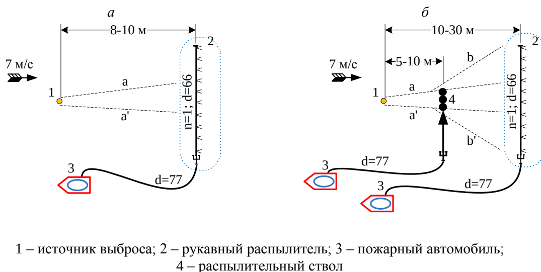
Рисунок –1. Схема постановки водяной завесы вблизи компактного источника выброса с использованием распылительного ствола
