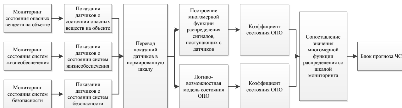
Рисунок –1. Структура мониторинга состояния объекта
