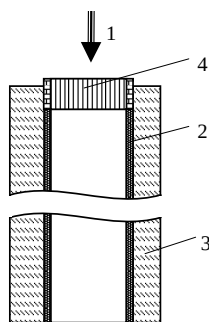
Рисунок – 2. Узел пиролиза: 1 – газовой поток, 2 – теплоизолированный канал, 3 – тепловая изоляция, 4 – устройство,
