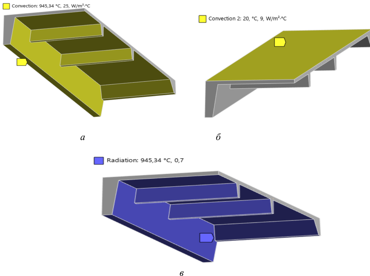
Рисунок 3. Прикладання граничних умов теплообміну досліджуваної залізобетонної порожнистої плити під час прикладання стандартного температурного режиму пожежі: а – конвекційний теплообмін обігрівної поверхні плити; б – конвекційний теплообмін у необігрівій поверхні плити; в – радіаційний теплообмін обігрівної поверхні плити.
