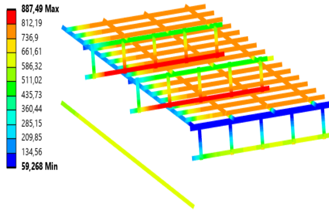
Рисунок 4. Розподіл температури по арматурі залізобетонній ребристої плиті під час впливу стандартного температурного режиму пожежі протягом 60 хв із використанням різних скінченно-елементних сіток: а – автоматична, б – за допомогою методу MultiZone, в – за допомогою методу Body Sizing.
