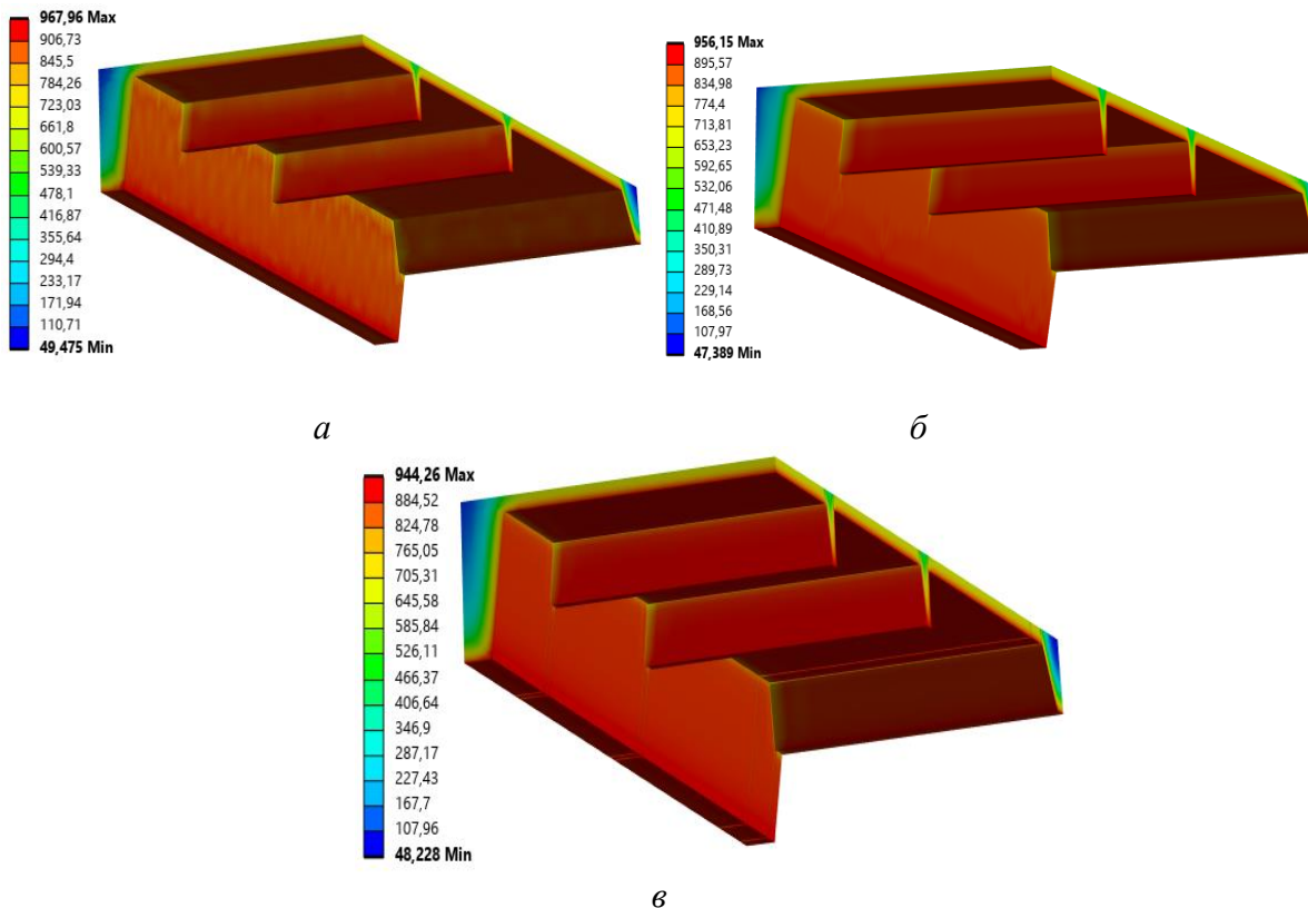
Рисунок 4. Розподіл температури по бетону залізобетонній ребристій плити під час впливу стандартного температурного режиму пожежі протягом 60 хв із використанням різних скінченно-елементних сіток: а – автоматична, б – за допомогою методу MultiZone, в – за допомогою методу Body Sizing.
