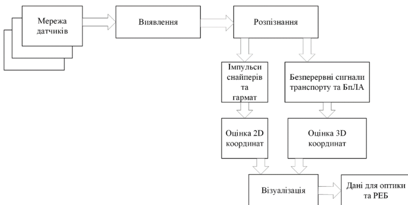
Схема 1. Структура акустичної системи локації
